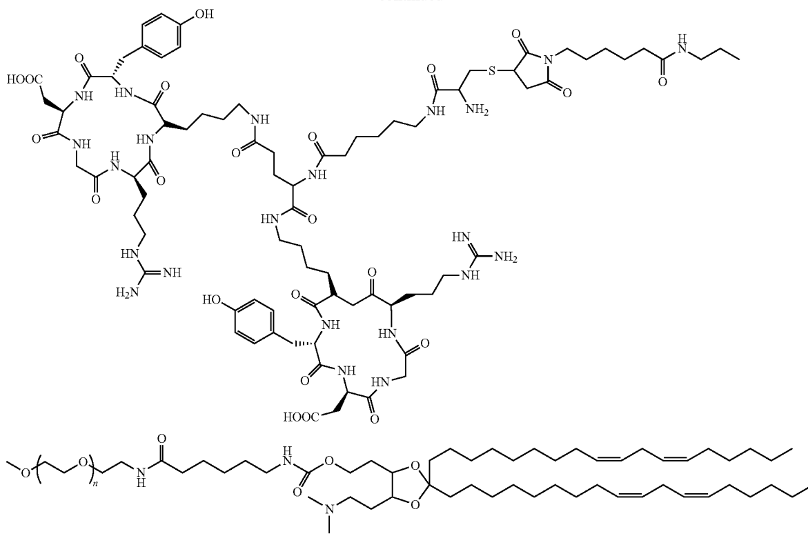
XTC 2 -RGD
