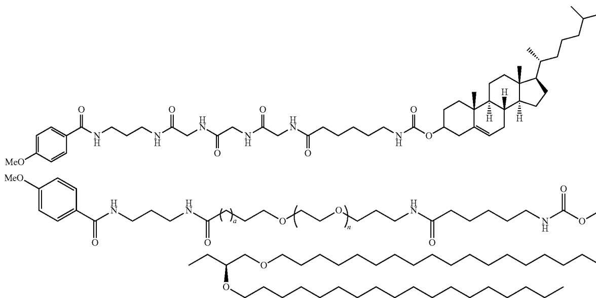
DSG-PEG-Anisamide
