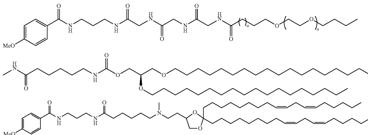
XTC 2 -Anisamide
