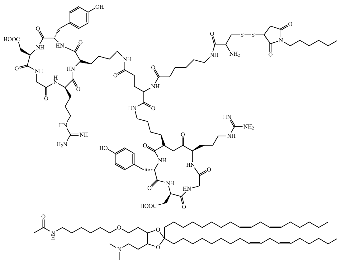
XTC 2 -RGD
