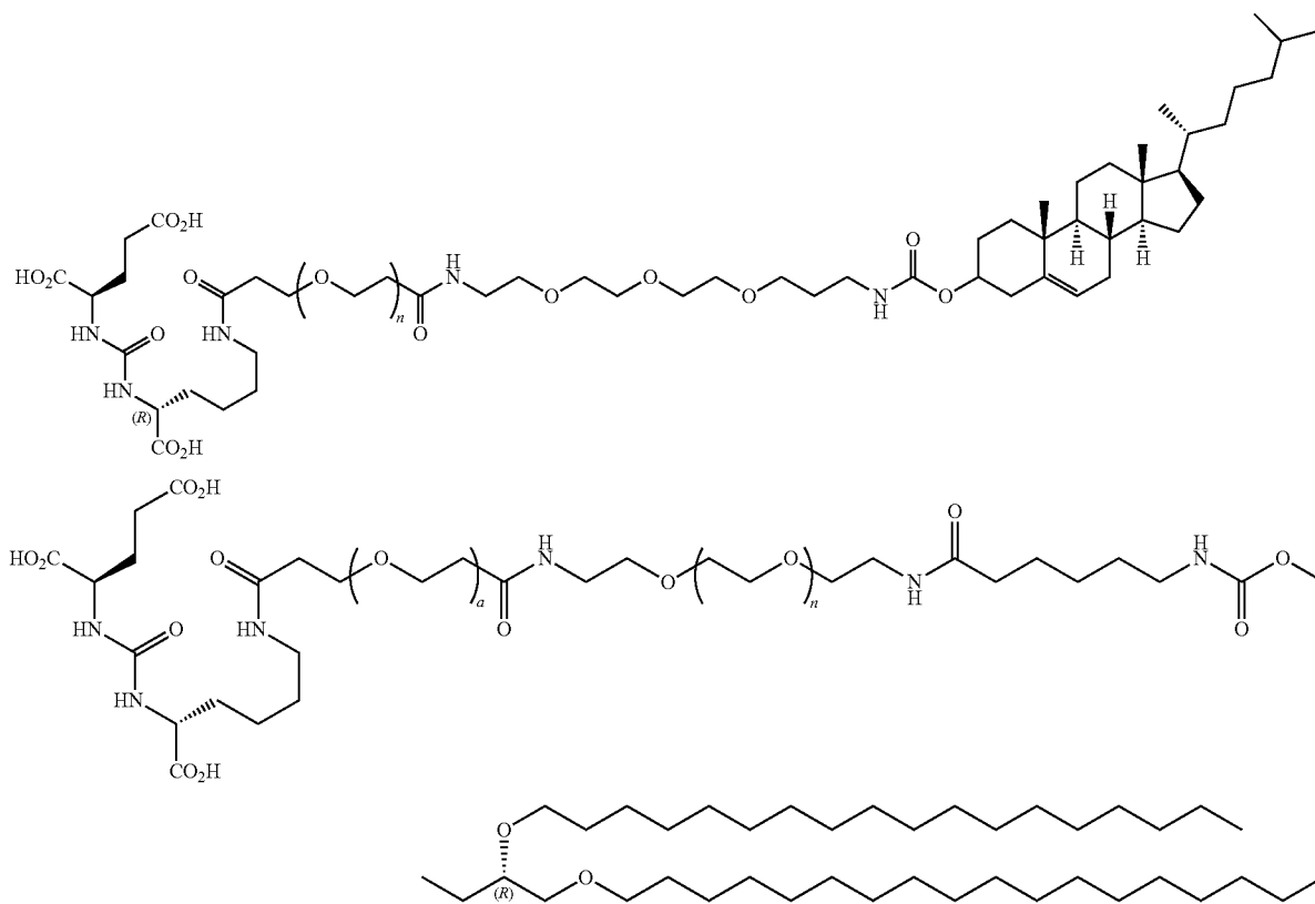
XTC 2 -RGD
