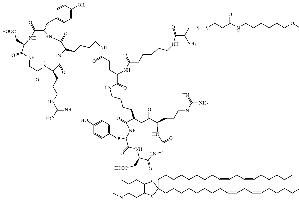
XTC 2 -RGD
