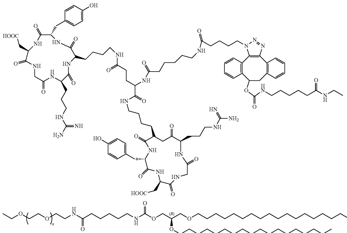
DSG-PEG-RGD
