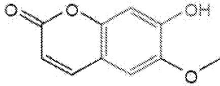
Scopoletin
