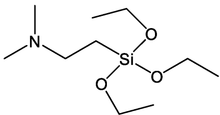
- (2-Dimethylaminoethyl)trimethoxysilan und
