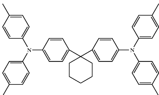
TPAC
