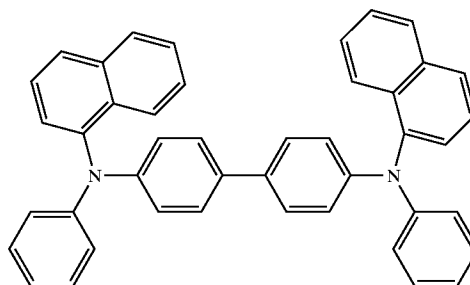
\alpha -NPD
