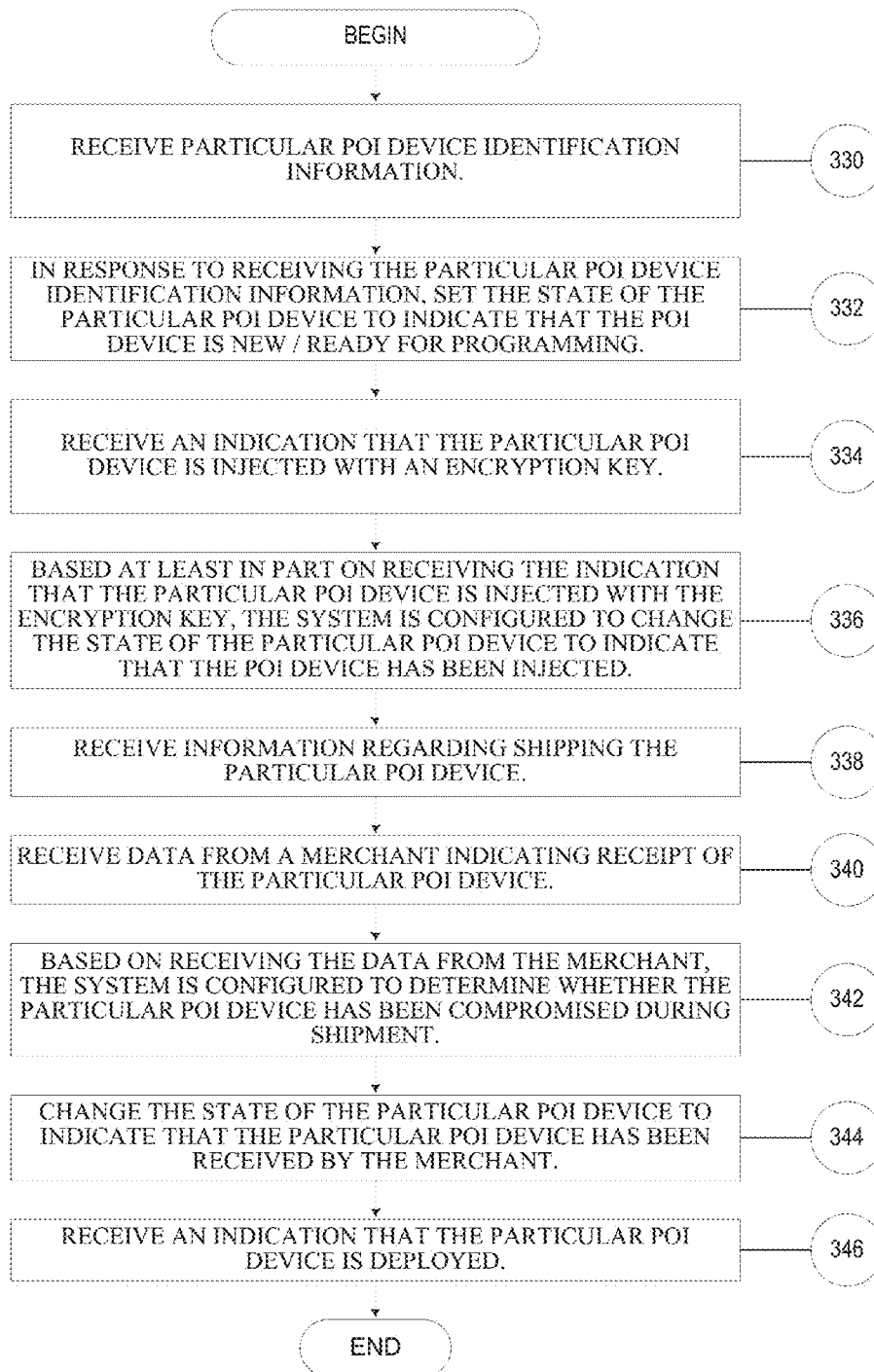
FIG. 3 EXEMPLARY POI HANDLING PROCESS
