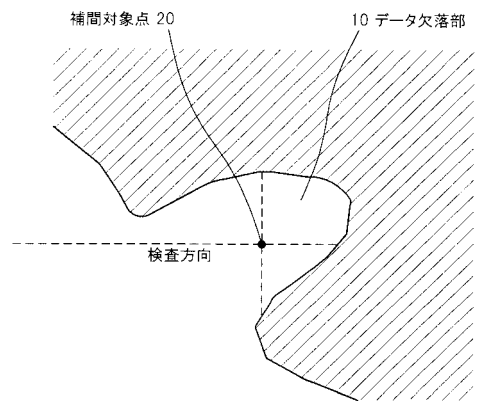
十字方向検査による補間対象点の検出の例
