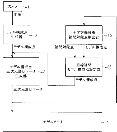
本発明による十字方向検査直線補間処理を加えた三次元形状モデル作製装置の例
