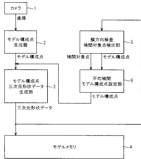
本発明による物体の三次元形状モデル作製装置の例
