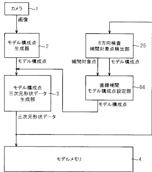
本発明による8方向検査直線補間処理を加えた三次元形状モデル作製装置の例
