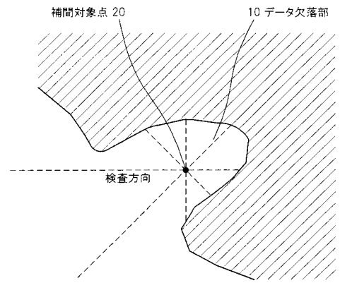
8方向検査による補間対象点の検出の例
