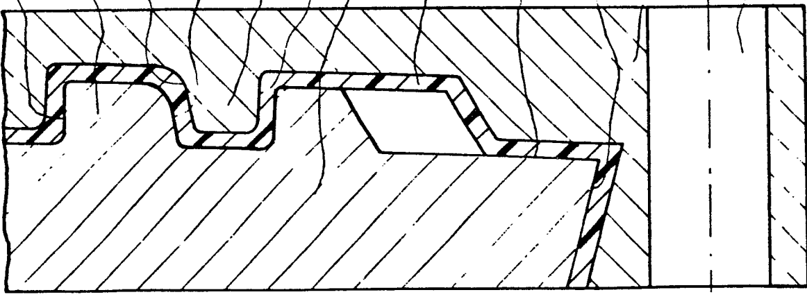
Fig. 3 Einzelheit X
