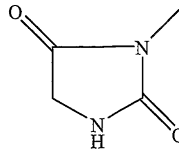
(hydantoin)
