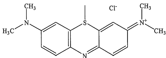
(methylene blue)
