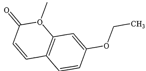
(7-ethoxycoumarin)
