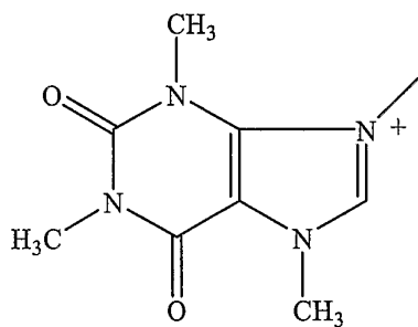
(caffeine)
