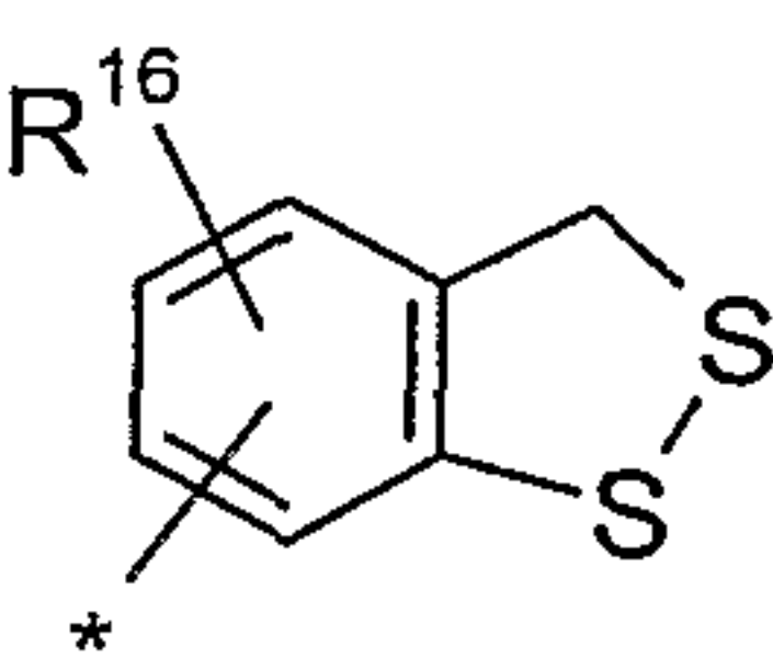
1,2-benzodithiolyl
