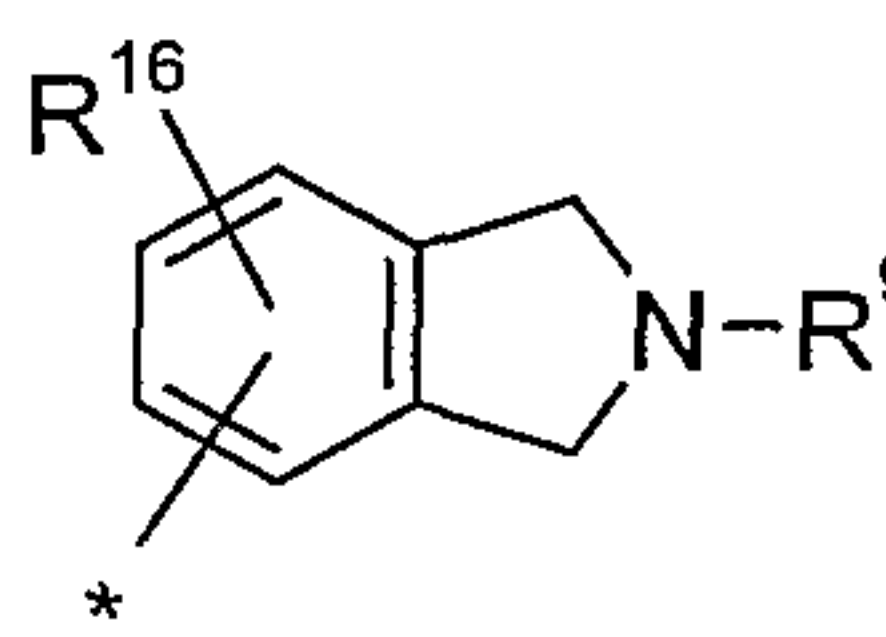
isoindoliny
