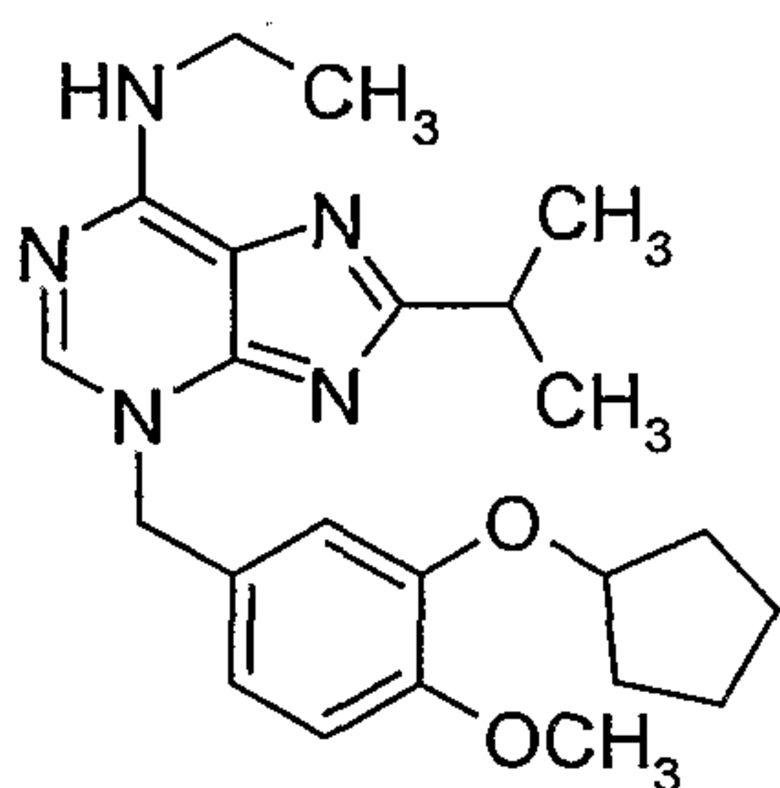
V-11294A (0.0.22)
