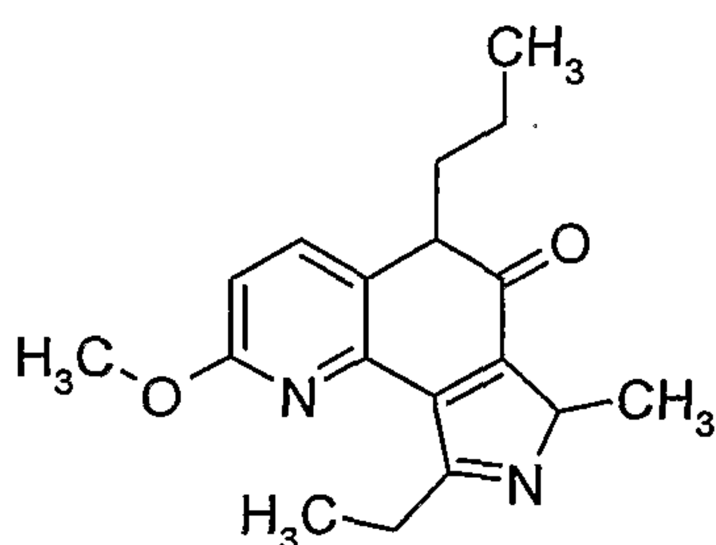
D-22888
