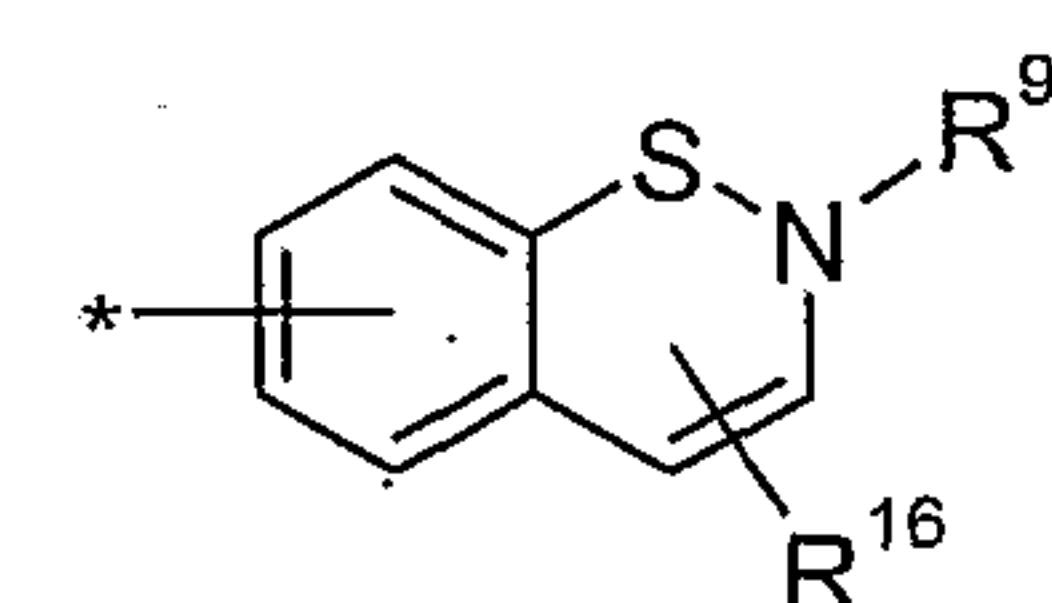
1,2-benzothiazinyl
