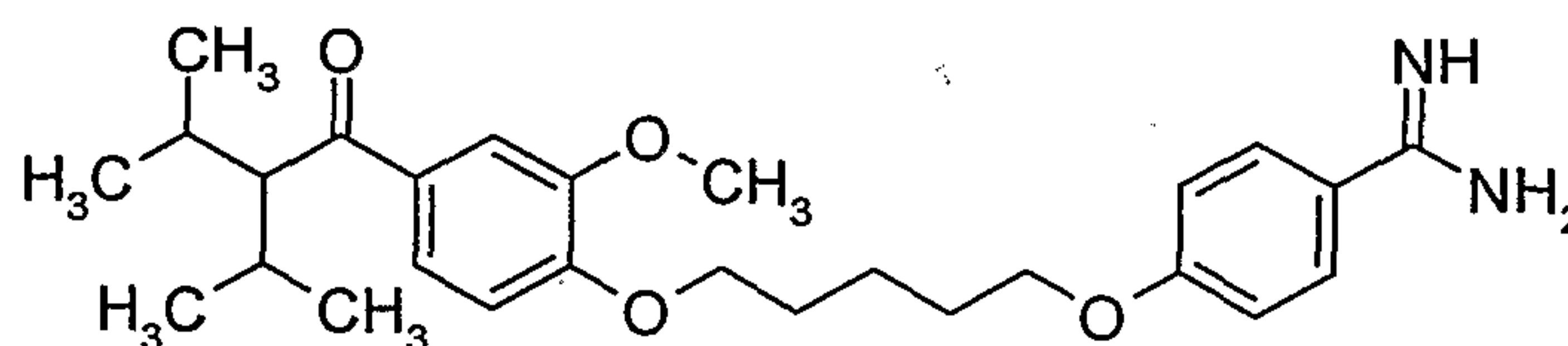
CGS-25019c (5.2.17)
