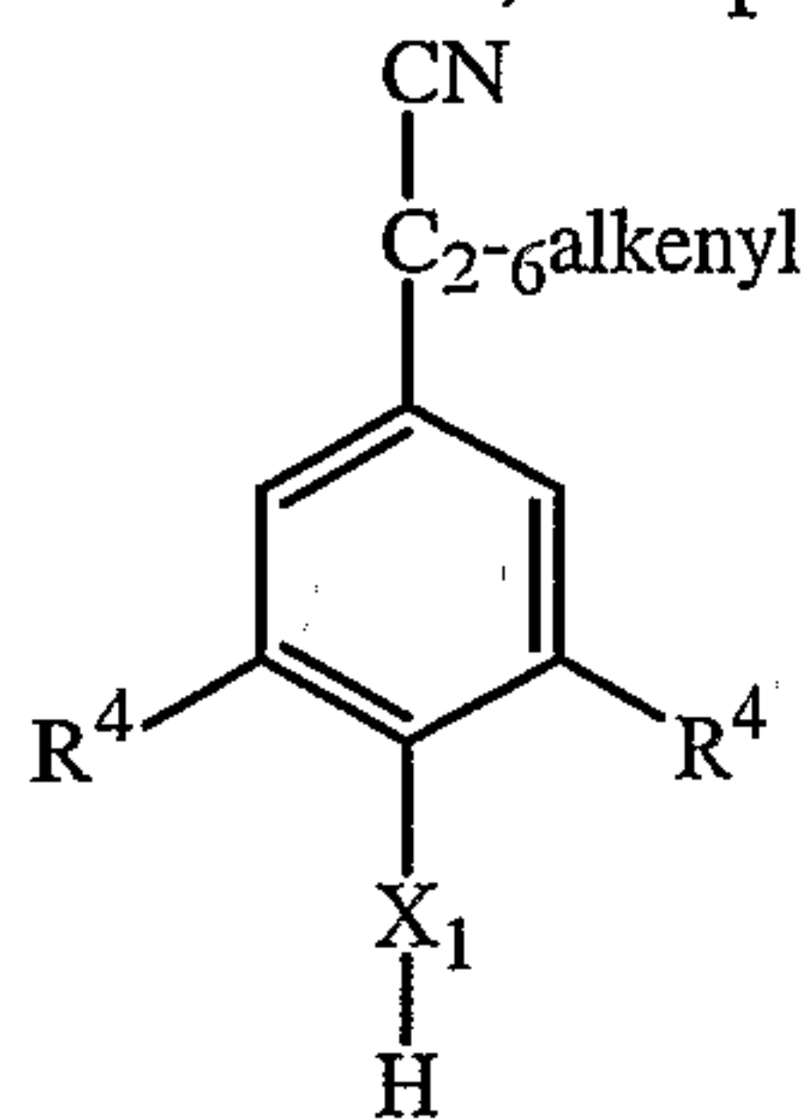
(III-b)
