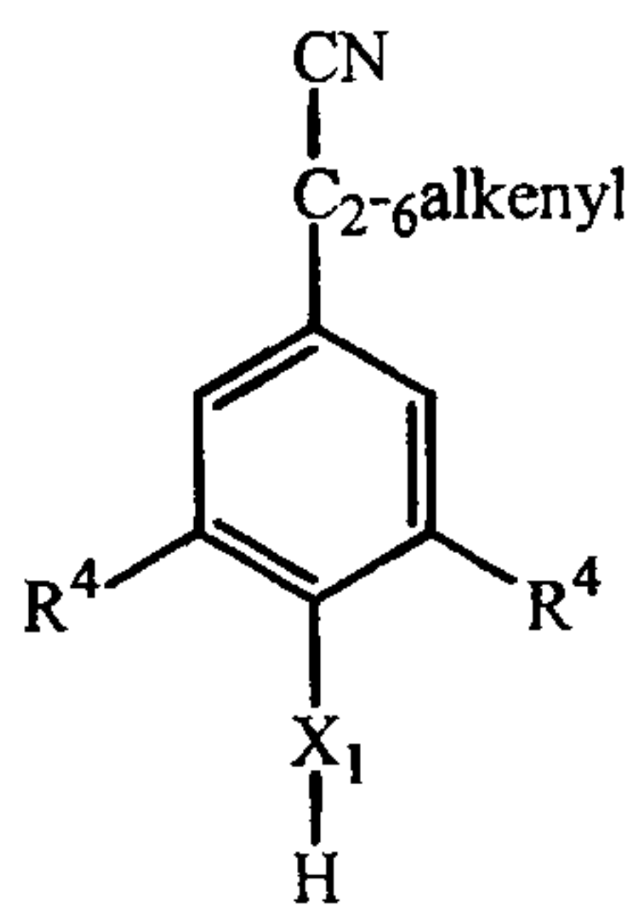
(III-b)
