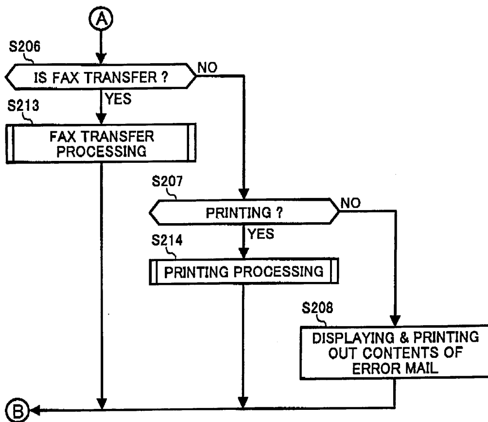
FIG. 32B
