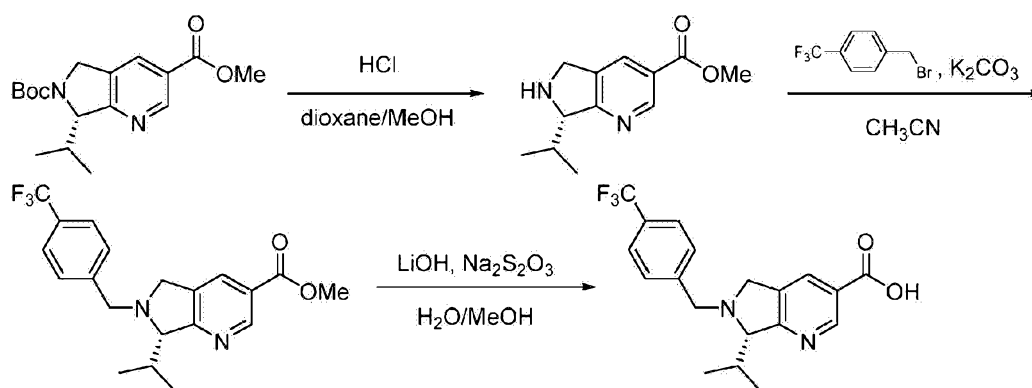
Scheme 14.
