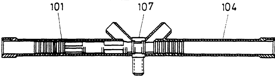
FIG. 17b
