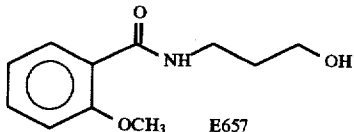
E657 3-(2-methoxybenzoylamino)-1-propanol
