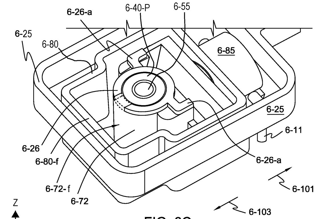
FIG. 6C
