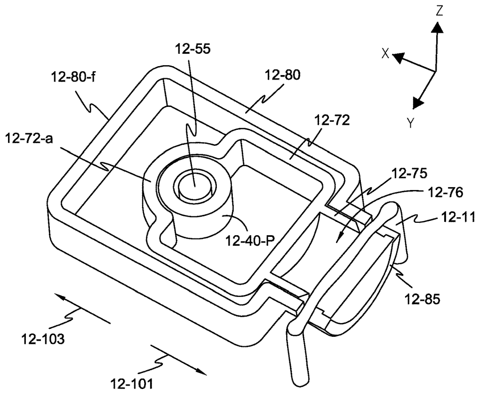
FIG. 12A
