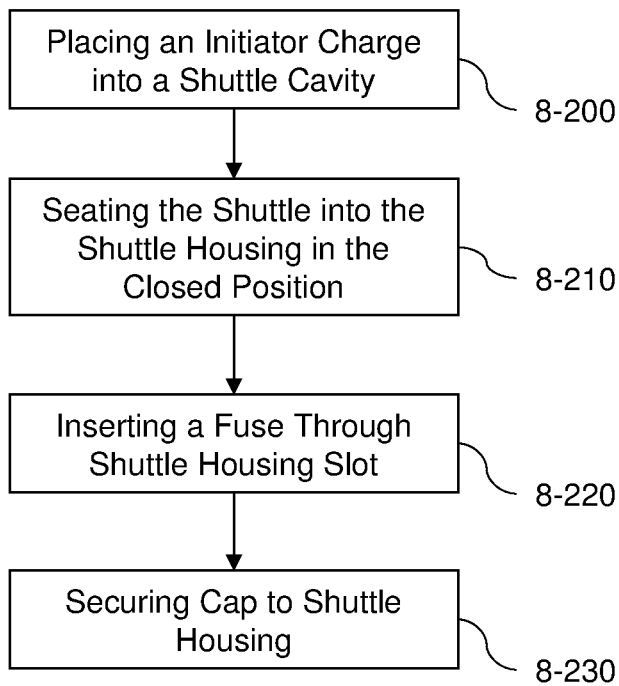
FIG. 8D
