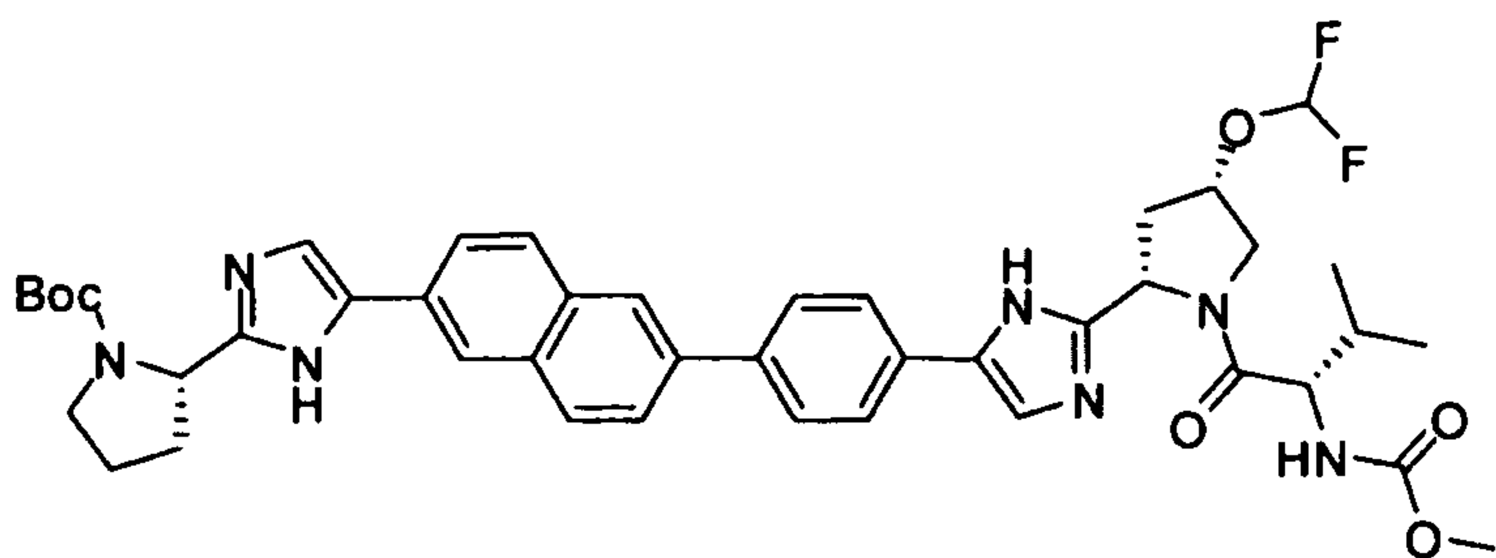
2-{5-[6-(4-{2-[4-Difluoromethoxy-1-(2-methoxycarbonylamino-3-methyl-butyl)-pyrrolidin-2-yl]-3H-imidazol-4-yl]-phenyl)-naphthalen-2-yl]-1H-imidazol-2-yl}-pyrrolidine-1-carboxylic acid tert -butyl ester
