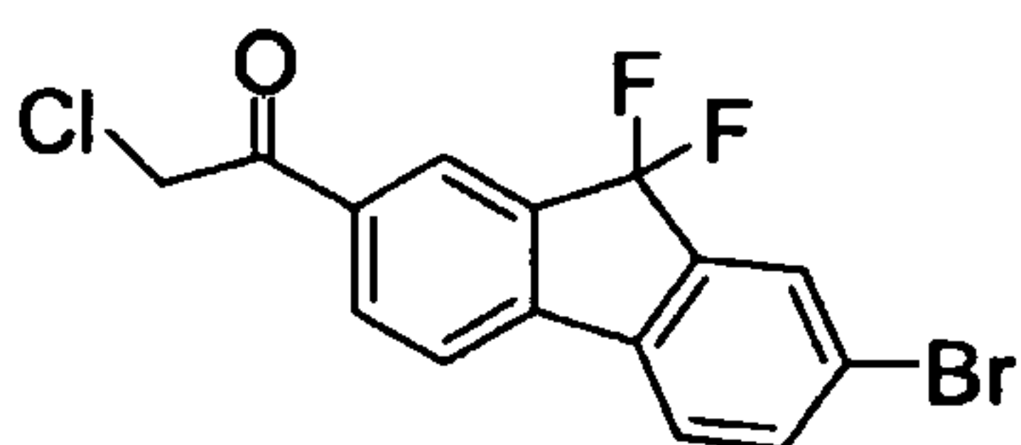
1-(7-Bromo-9,9-difluoro-9H-fluoren-2-yl)-2-chloro-ethanone
