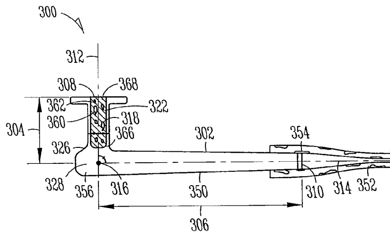
SECTION 3B-3B
