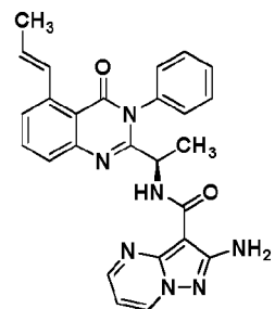
Compound 2070r,
