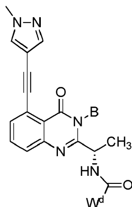
XIII.
