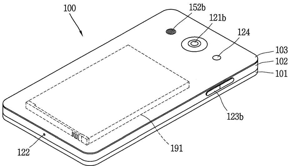
도면1c
