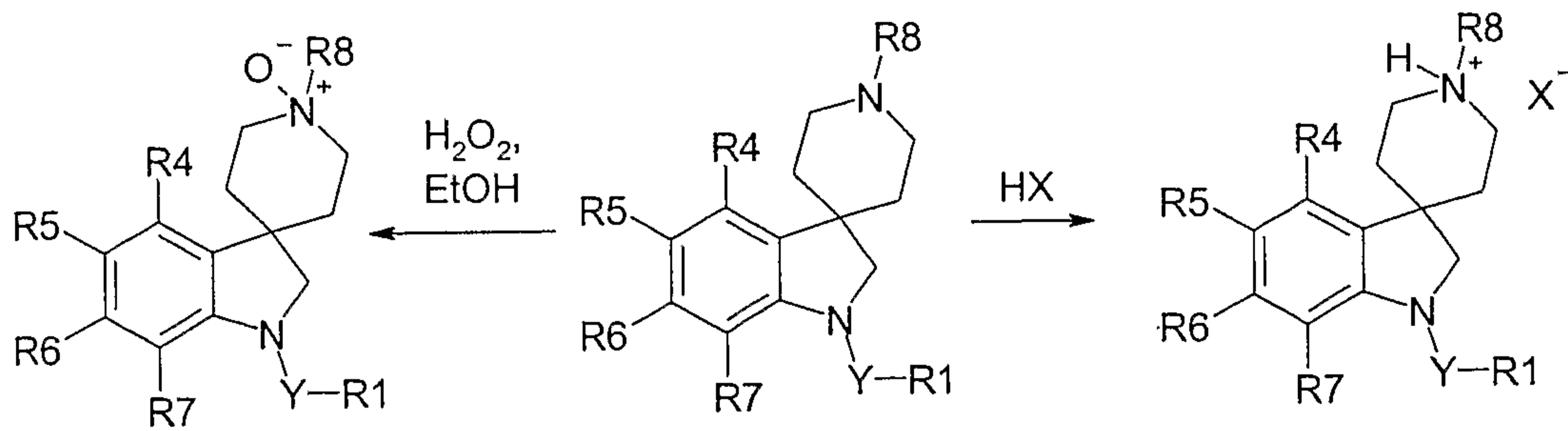
SCHEME VI
