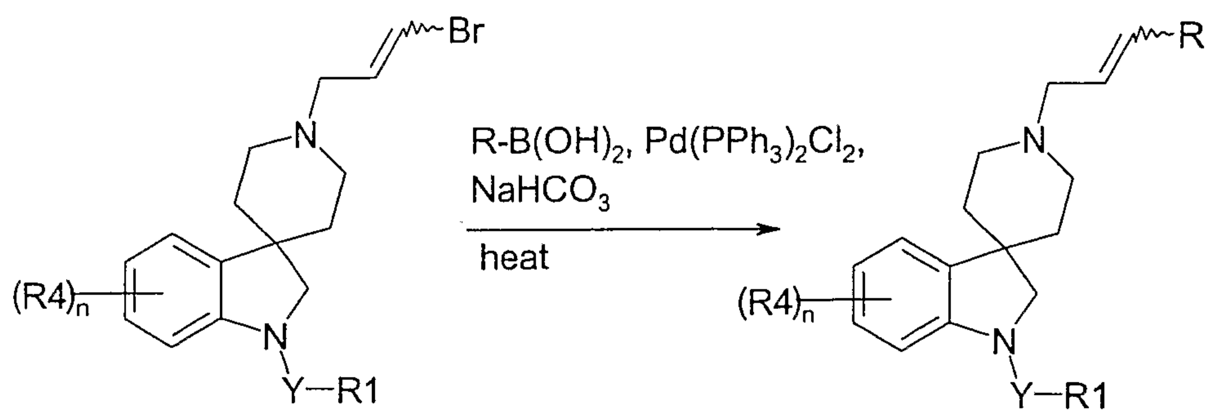
Scheme VA
