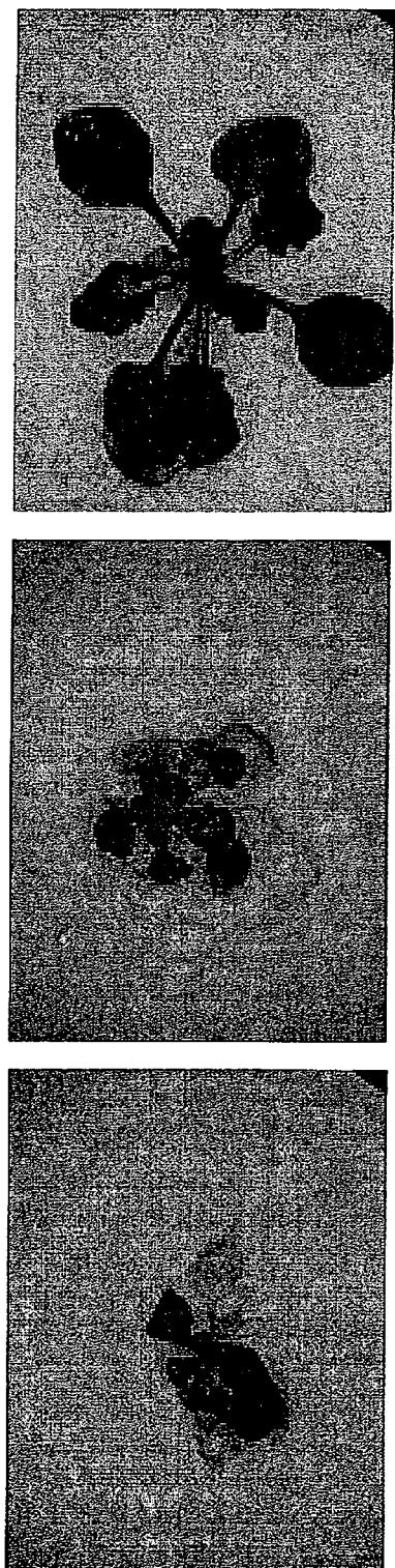
PpMYB-1
