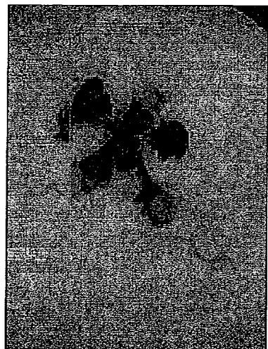
PpAPS-2
