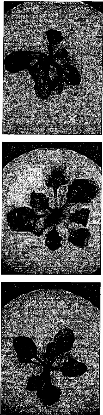
PpSFL-1
