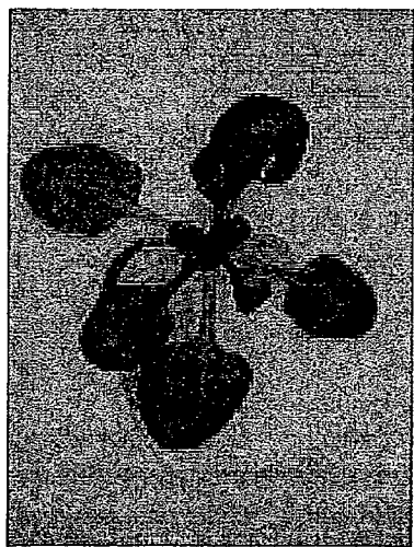
PpZF-3
