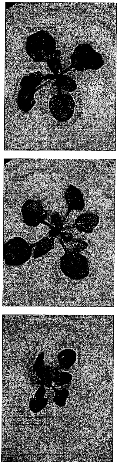
PpCABF-3
