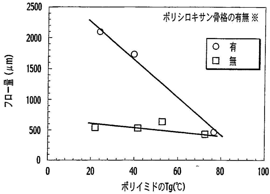
使用ポリイミドのTgとフィルムのフロー量との関係
