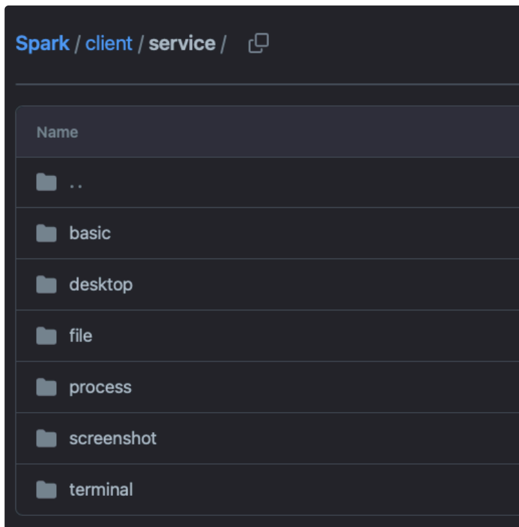
SparkRAT Capabilities
