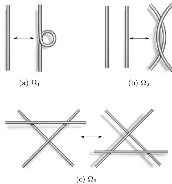
Abbildung 1.12: Reidemeister-Züge
