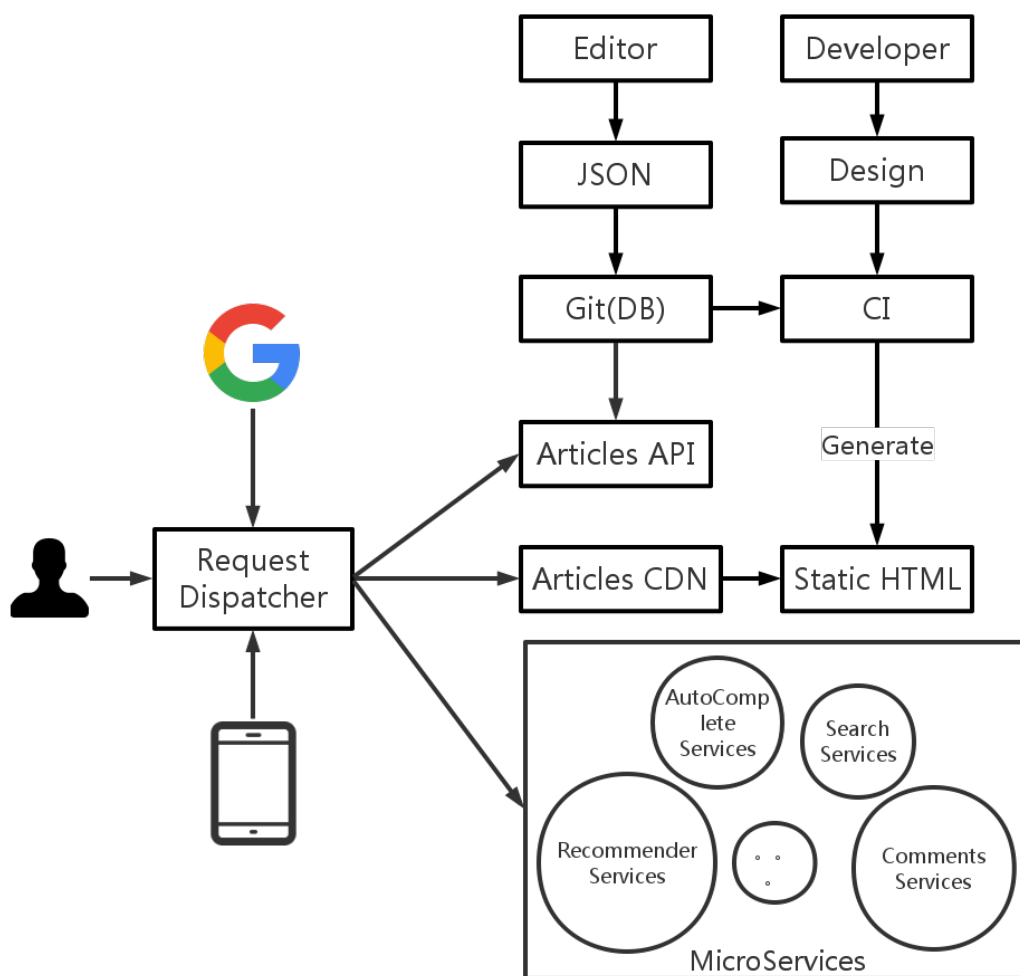
图 115: CQRS 结合微服务
