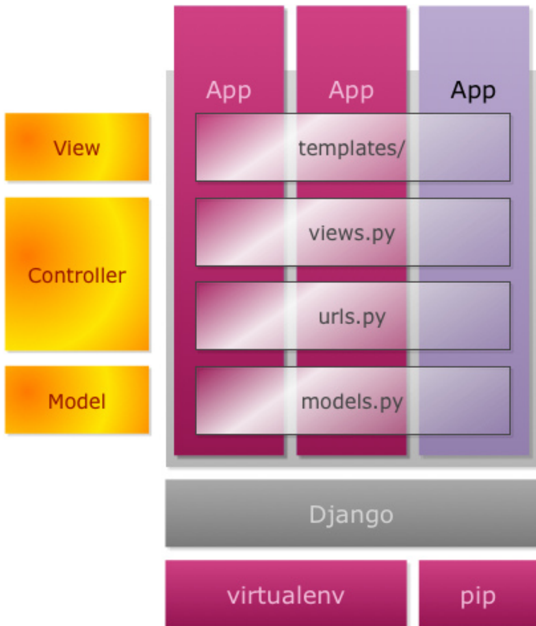
图 103: Django APP 架构
