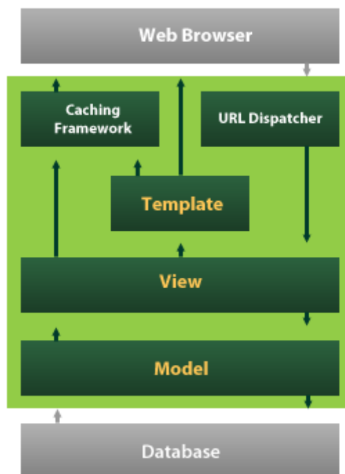
图 101: Django MTV 架构
