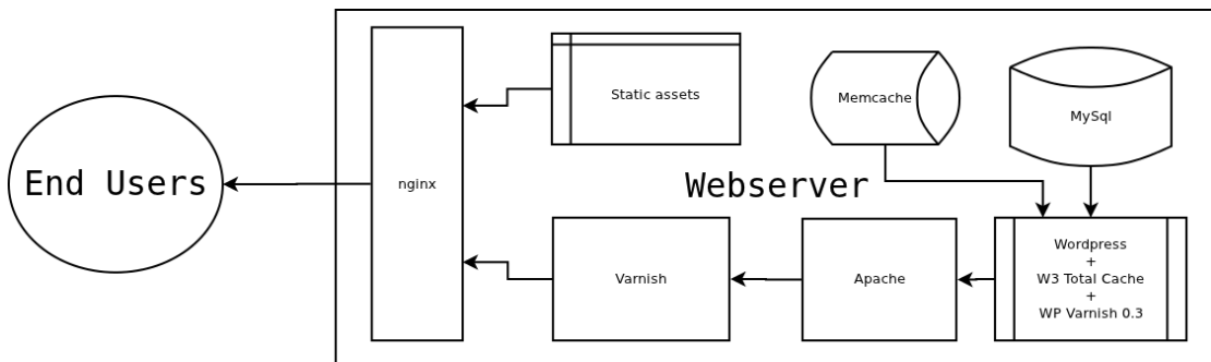
图 107: 带缓存的 Web 架构
