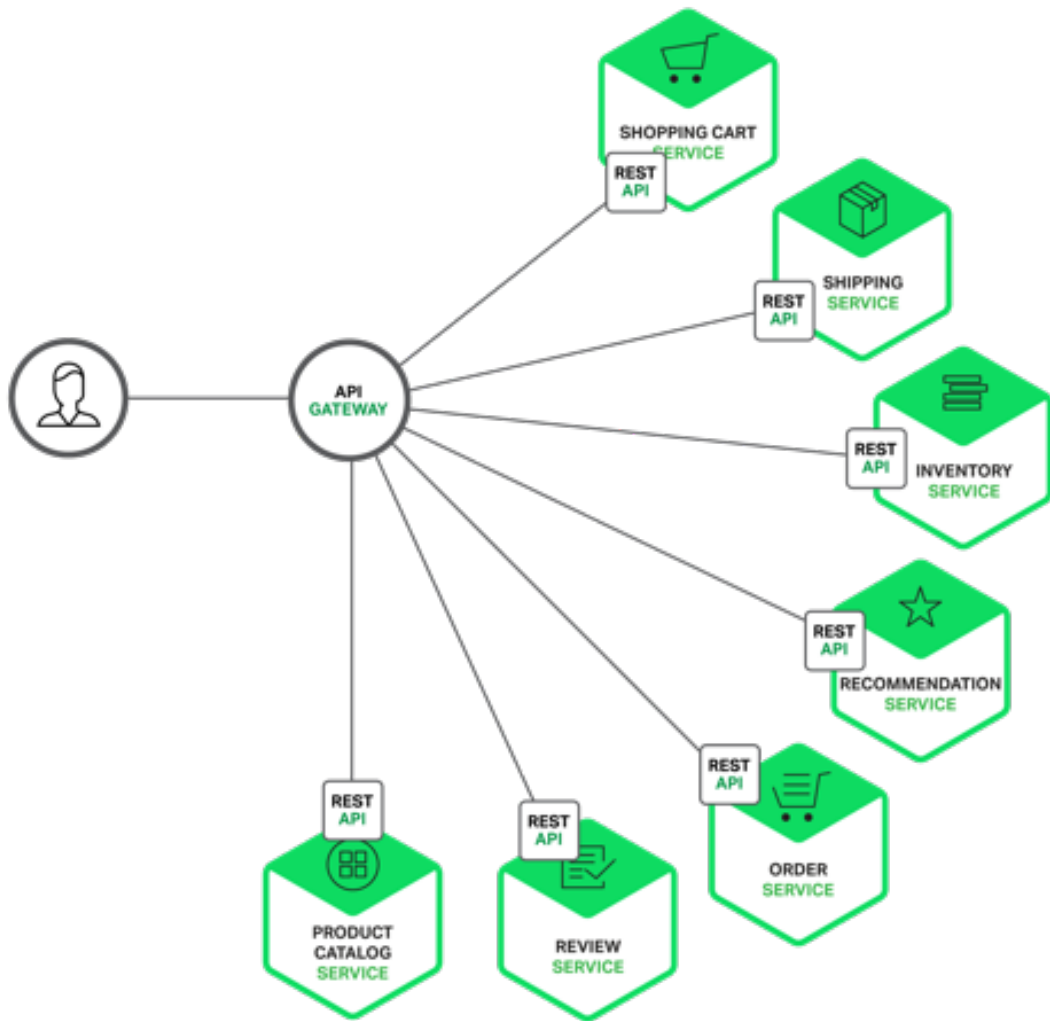
图 114: Nginx 解耦微服务
