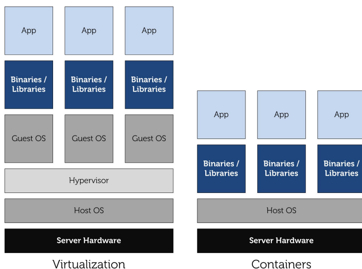
图 55: LXC vs VM
