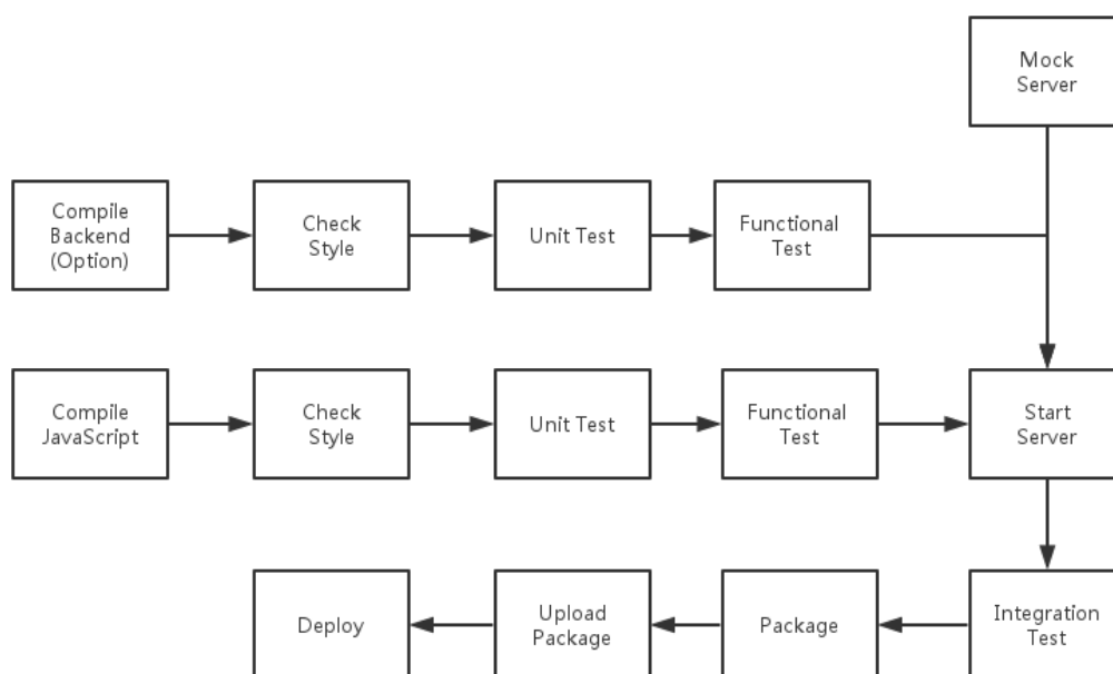
图 43: 构建过程
