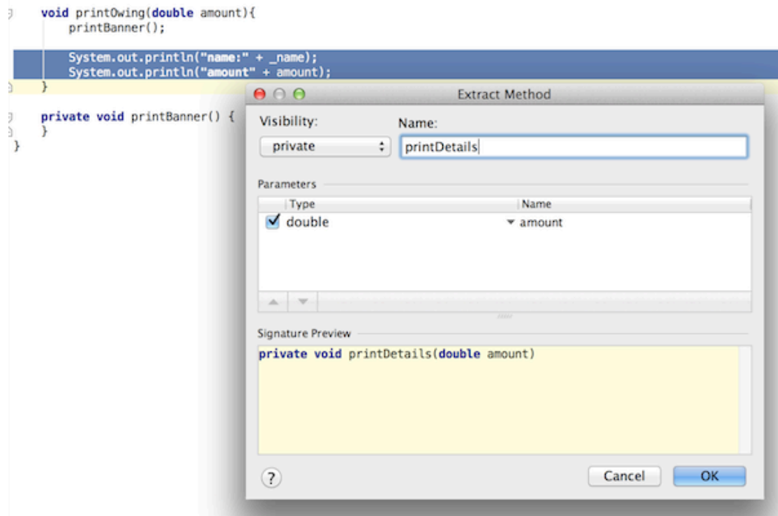
图 50: Extrect Method
