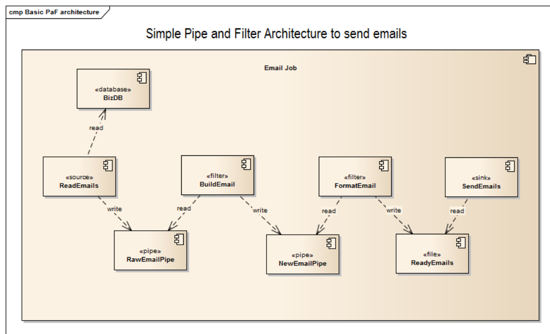
图 94: 发送邮件中的 Pipe and Filters 模式
