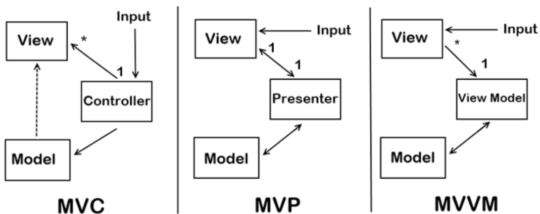
图 32: MVC、MVVM、MVP 对比
