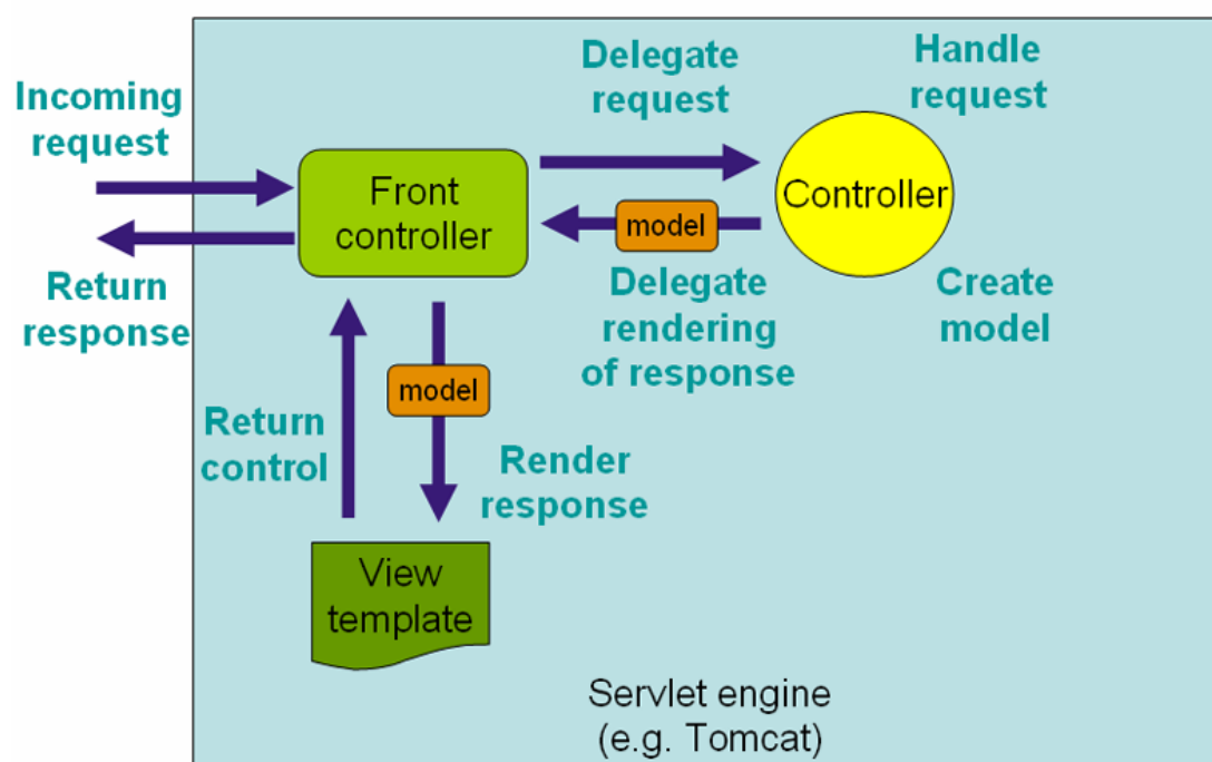
图 93: Spring MVC
