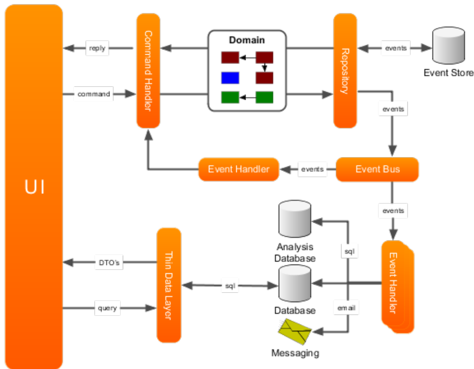
图 113: CQRS 和 EventBus
