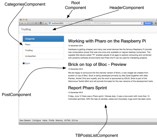
Figure 5-8 Les composants composant l'application TinyBlog (en mode non admin).
