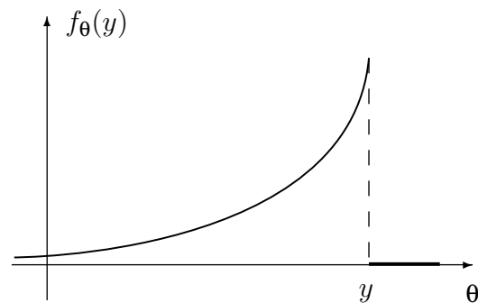
Рис. 6. Плотность в примере 19
