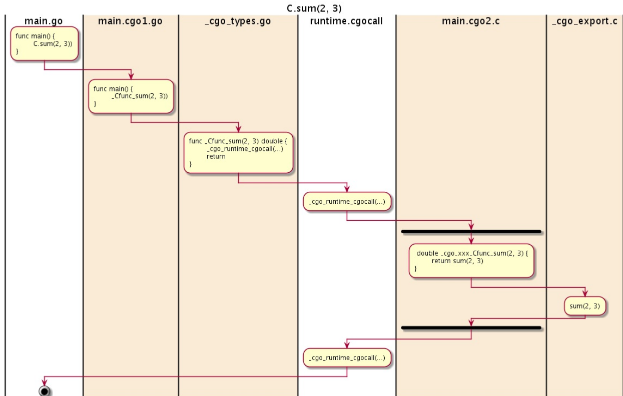
图 2.5-2 调用C函数
