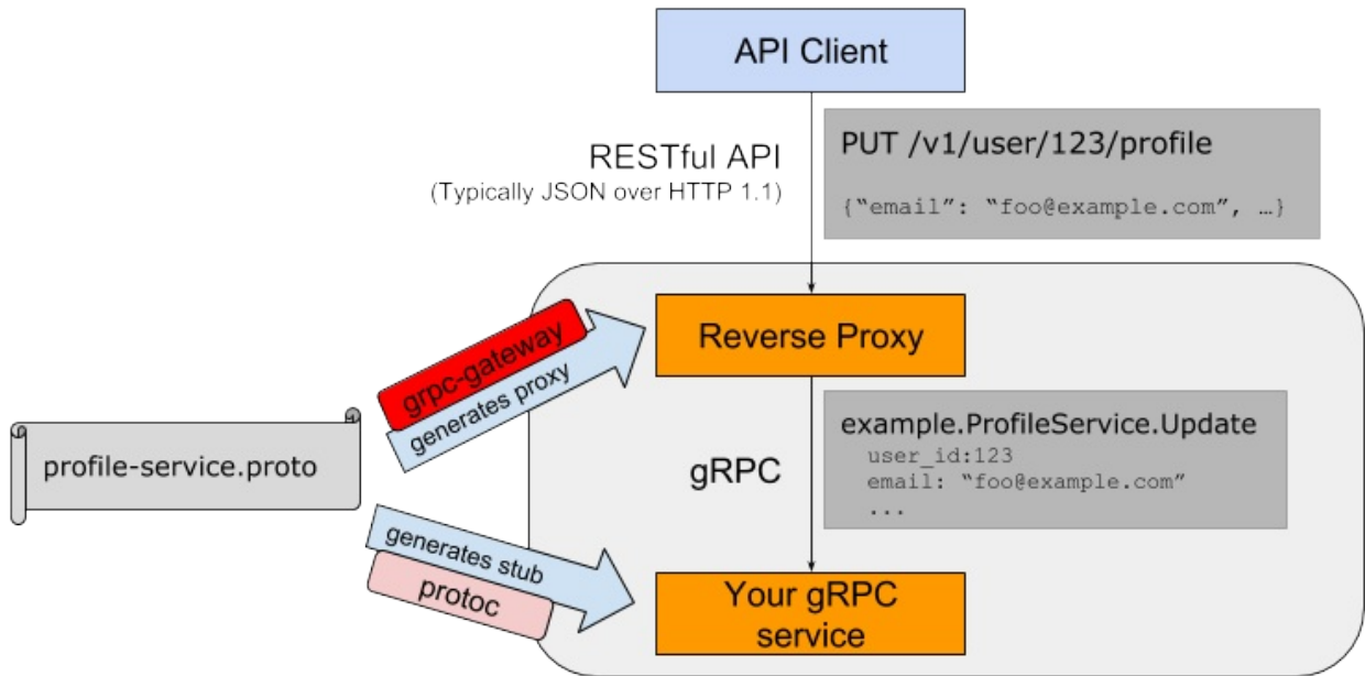
图 4.6-1 Grpc-Gateway工作流程
