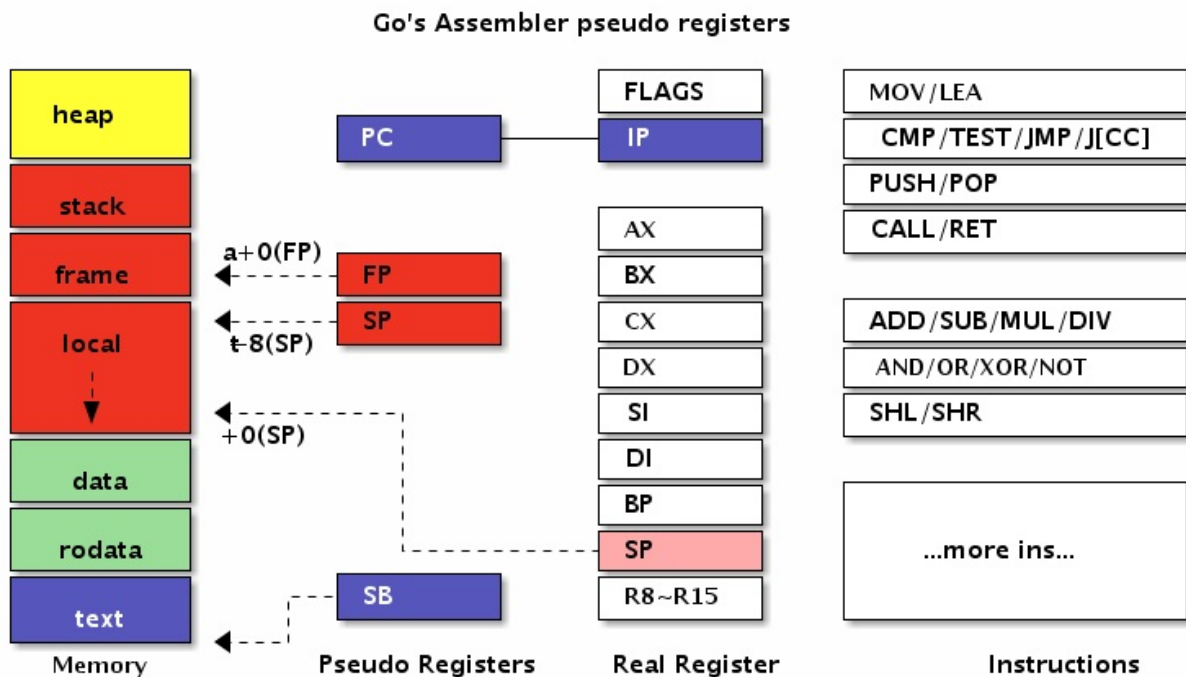
图 3.2-3 Go汇编的伪寄存器
