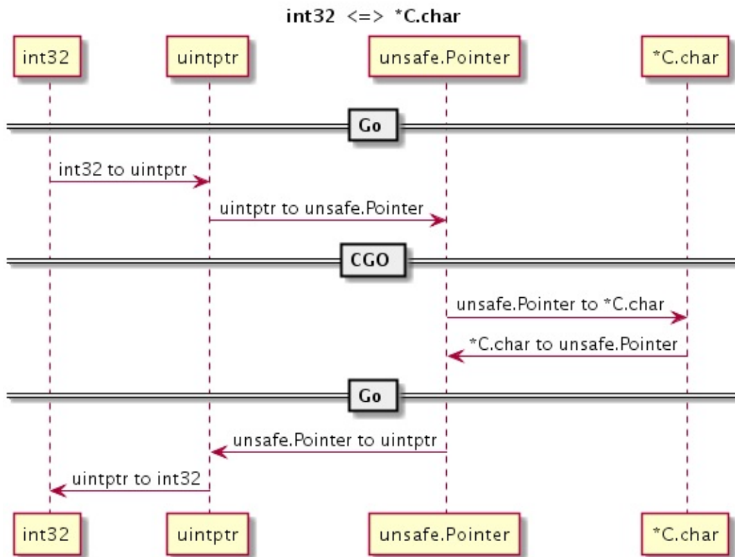
图 2.3-2 int32 和 *char 指针转换*
