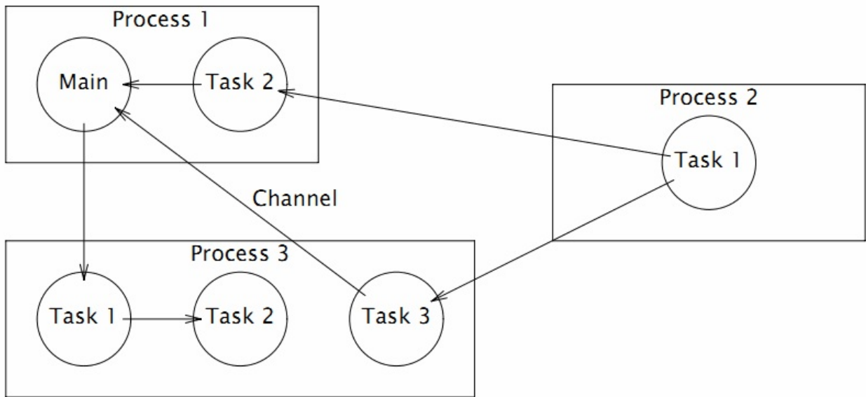
图 1.2-3 Alef并发模型
