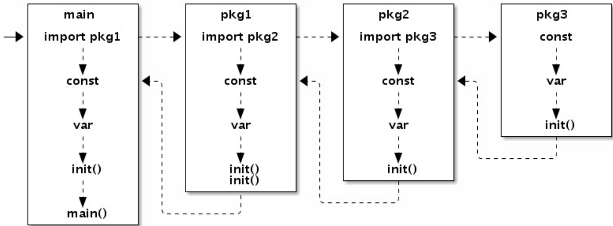
图 1.5-1 包初始化流程
