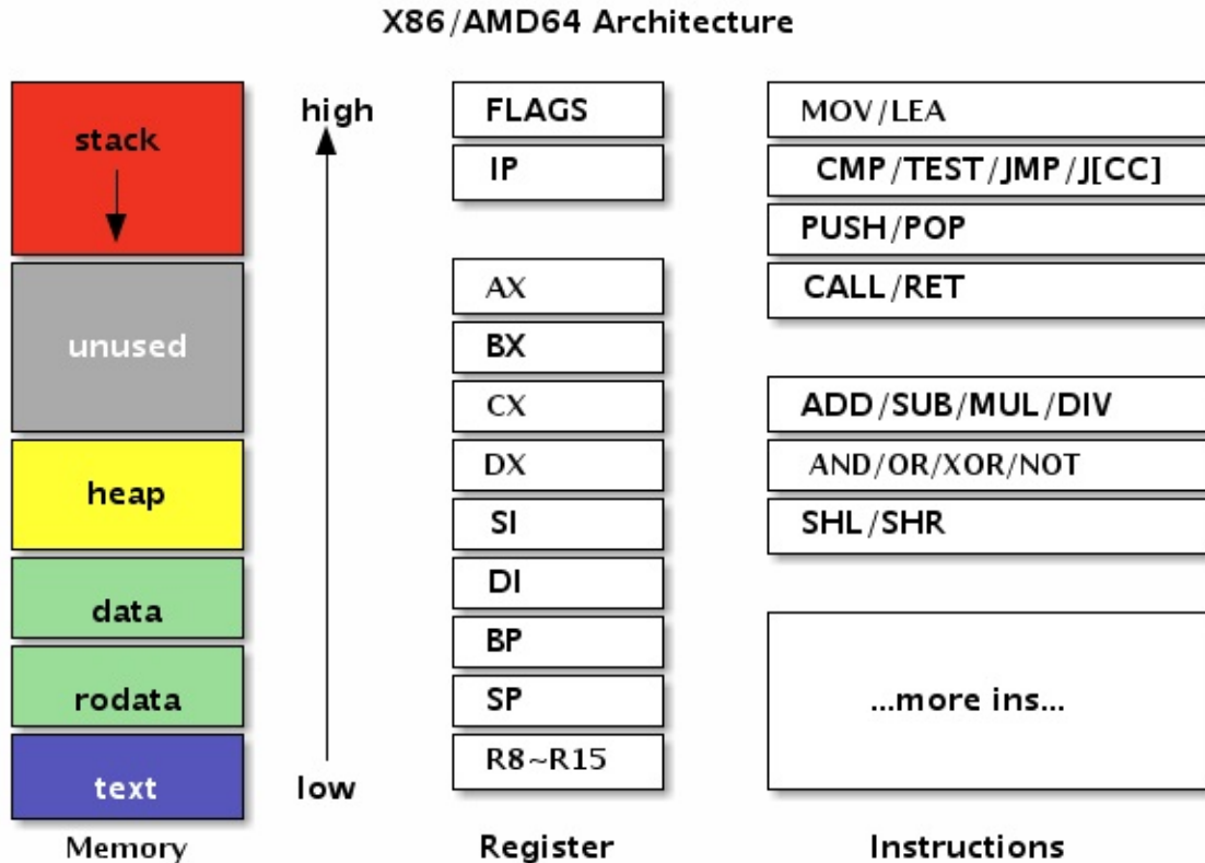
图 3.2-2 AMD64架构
