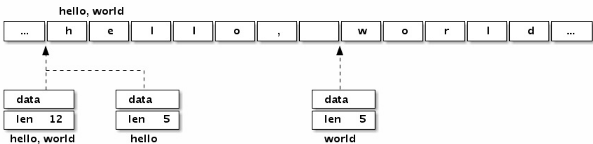
图 1.3-2 字符串布局
