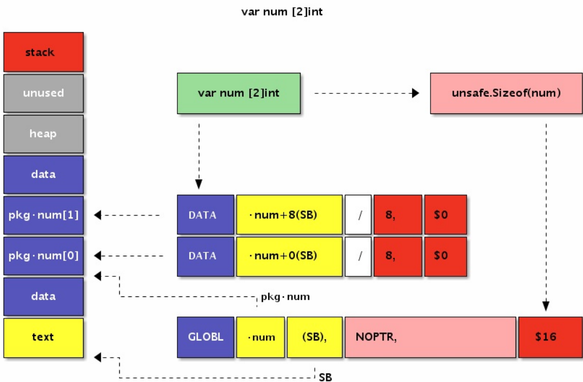
图 3.3-3 变量定义
