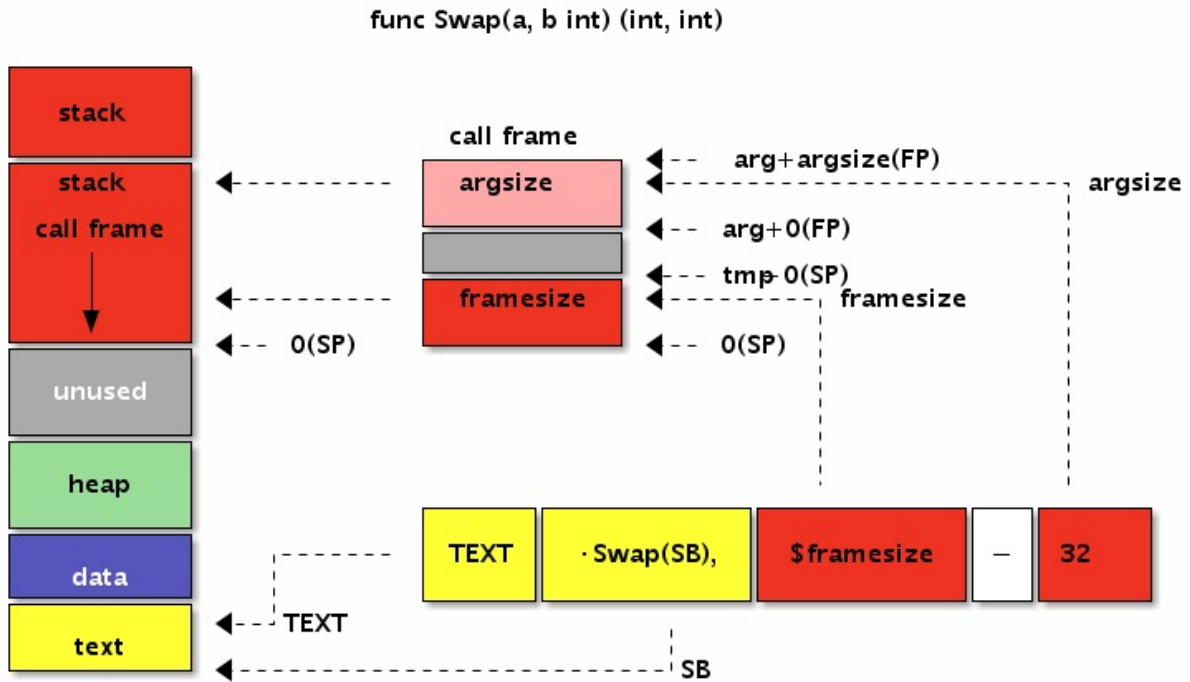
图 3.4-2 函数定义
