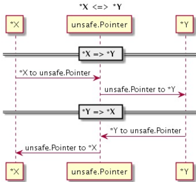
图 2.3-1 X类型指针转Y类型指针
