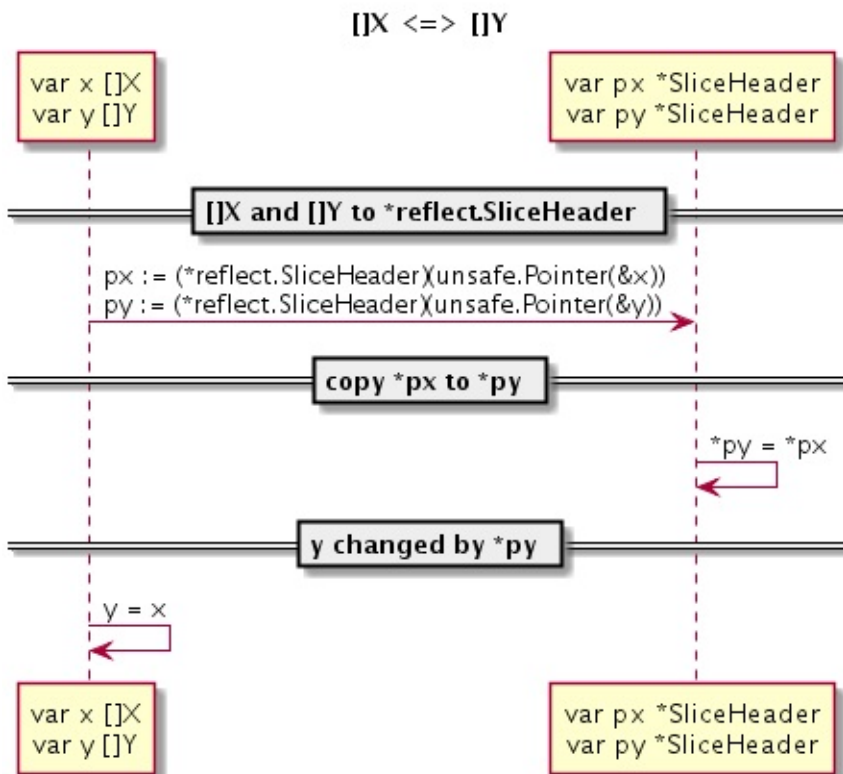
图 2.3-3 X类型切片转Y类型切片
