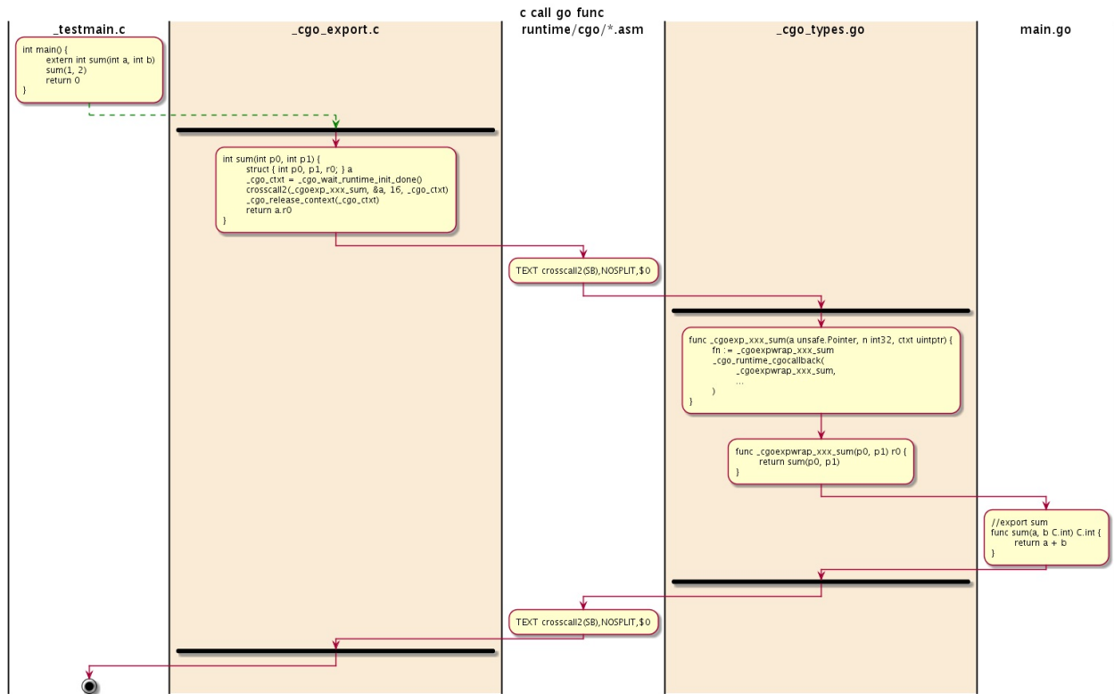
图 2.5-3 调用导出的Go函数
