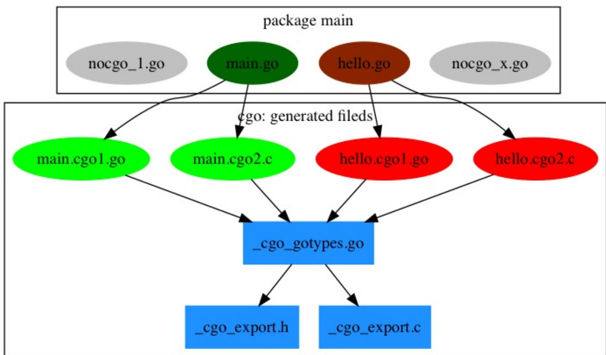
图 2.5-1 cgo生成的中间文件
