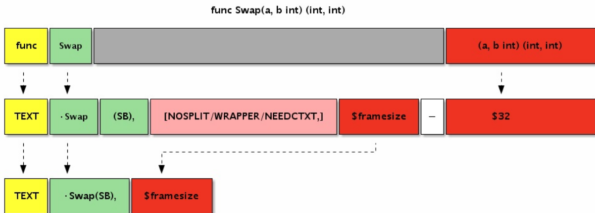
图 3.4-1 函数定义
