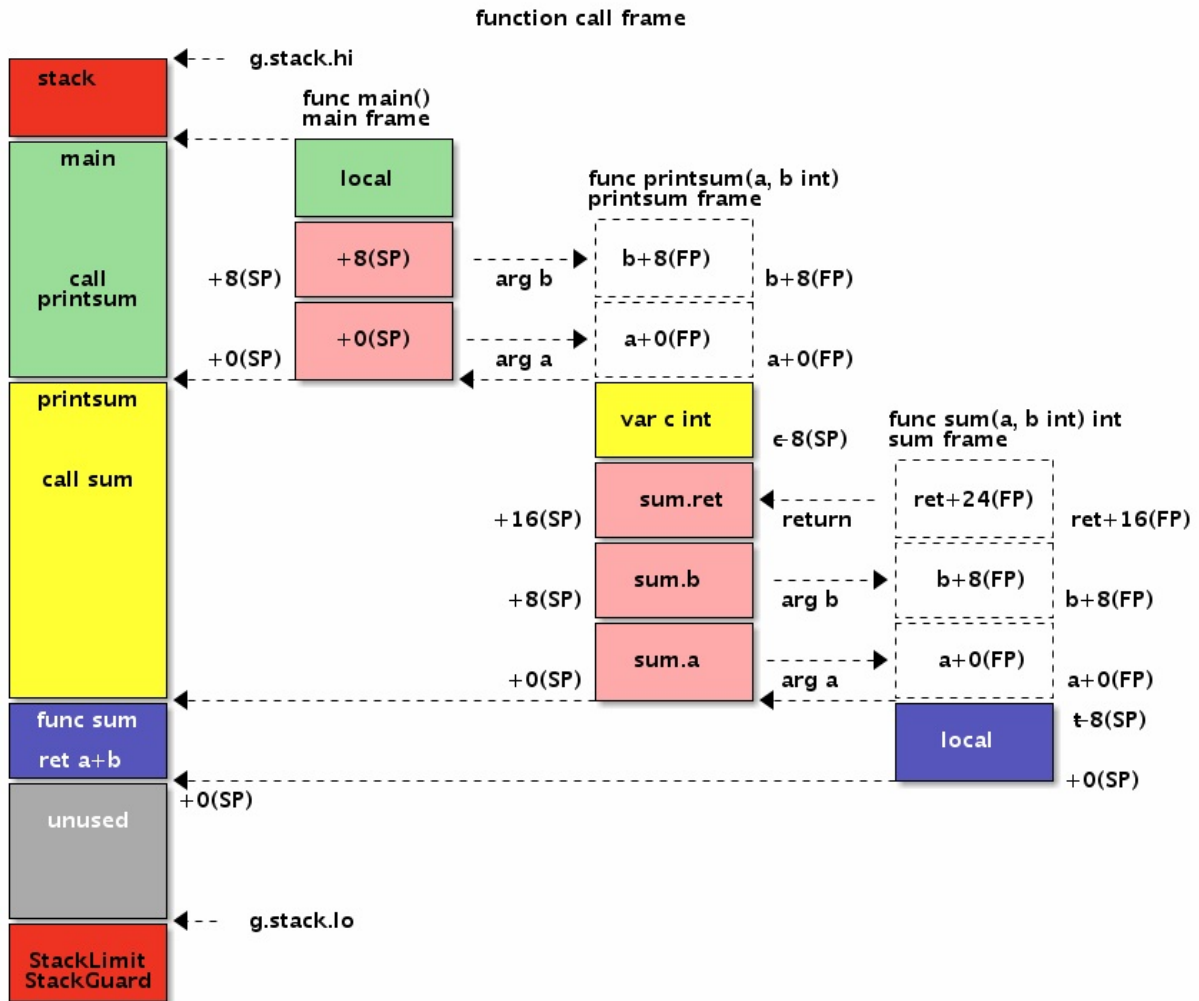
图 3.4-5 函数帧
