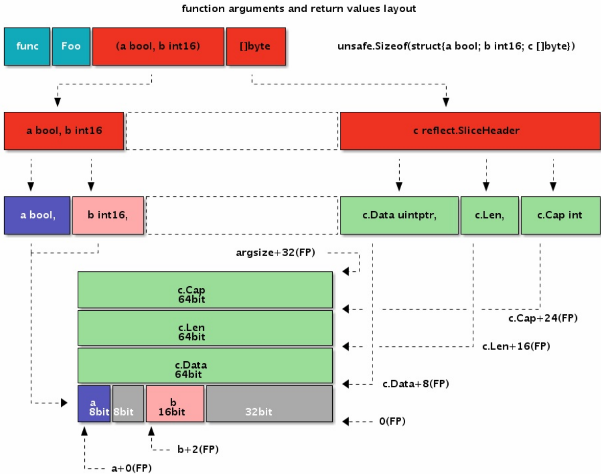
图 3.4-3 函数的参数
