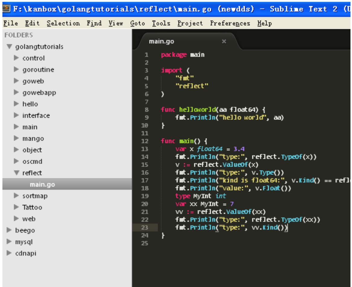
图1.6 sublime项目管理界面
