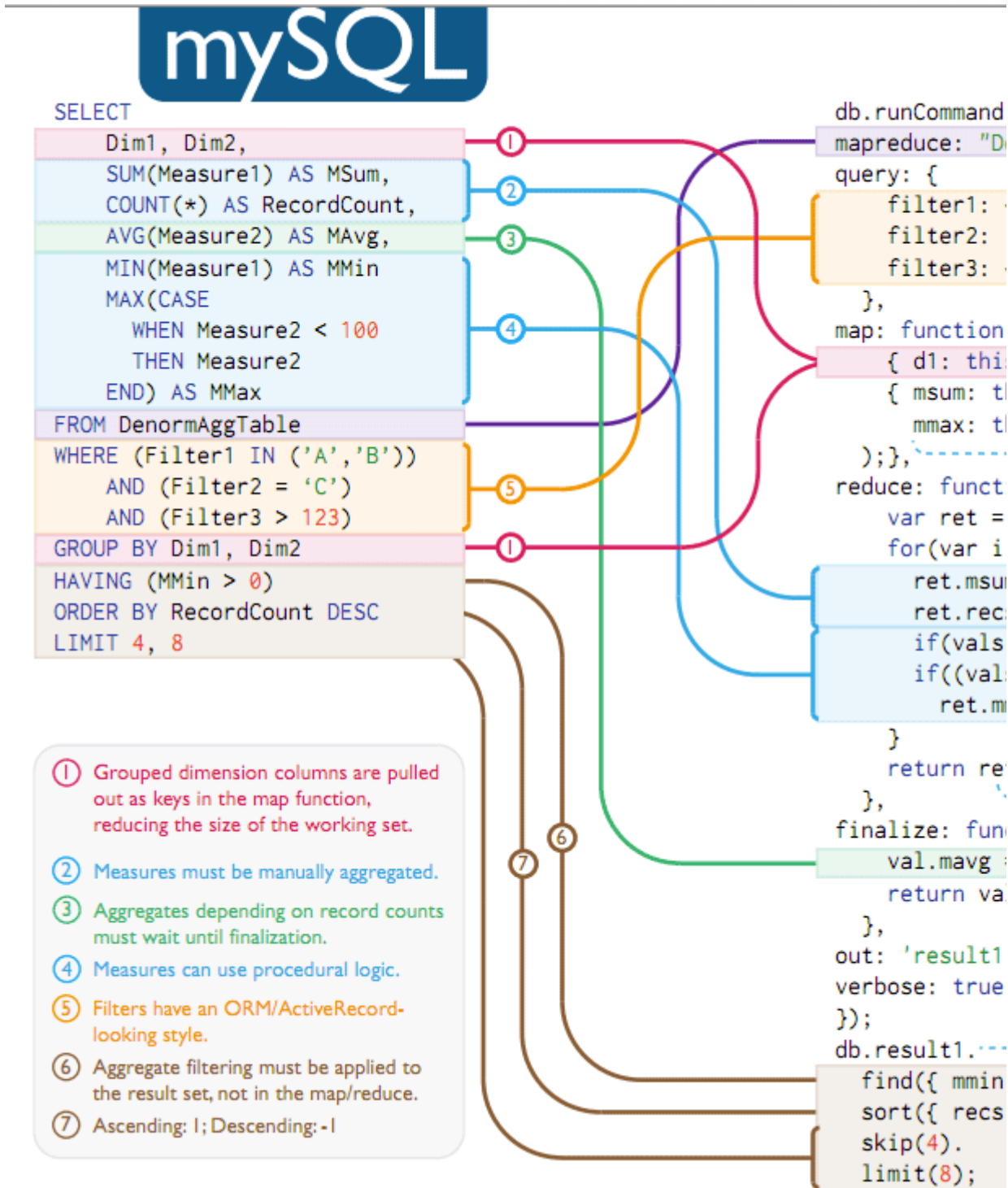
图5.1 MongoDB和Mysql的操作对比图
