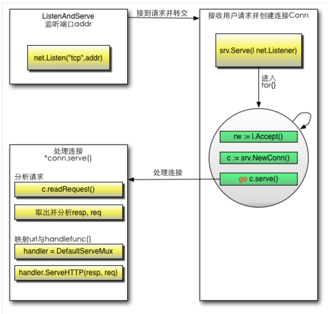
图3.10 一个http连接处理流程
