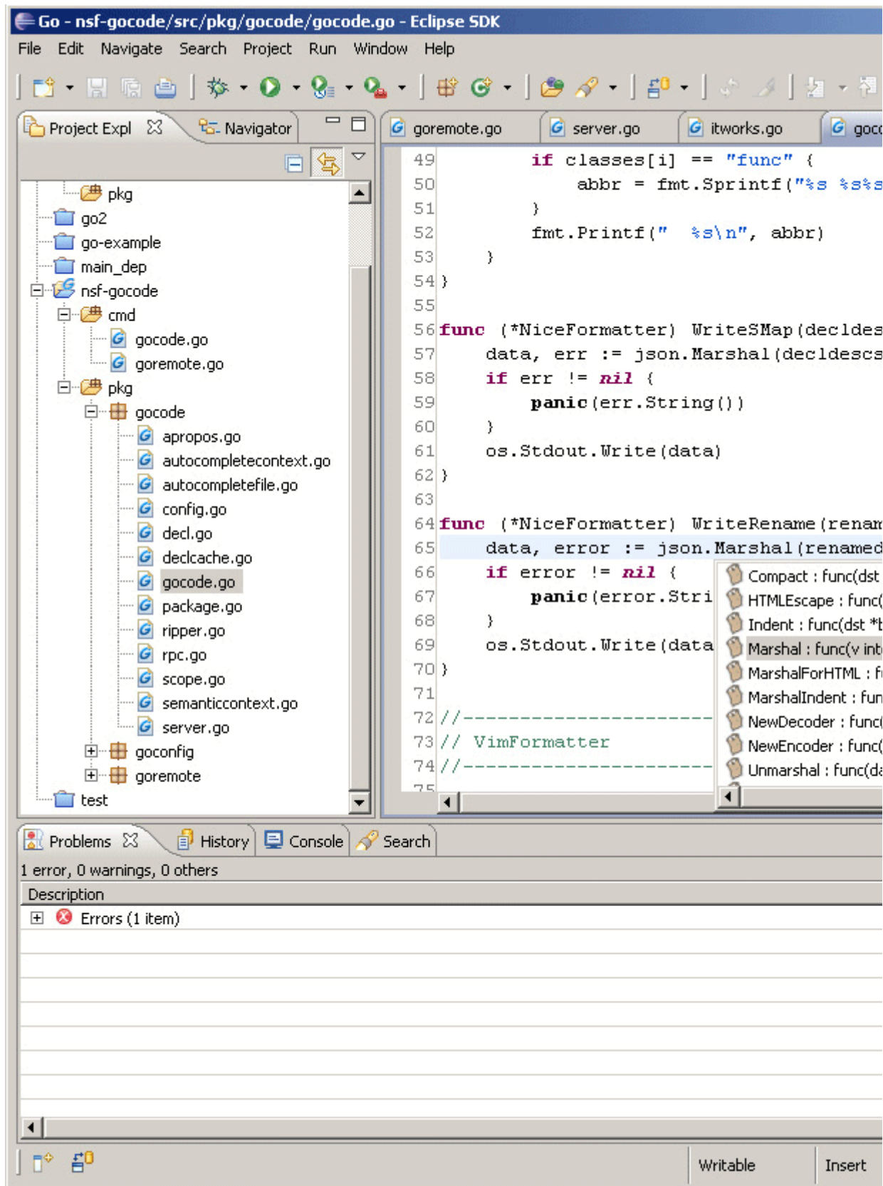
图1.11 Eclipse编辑Go的主界面
