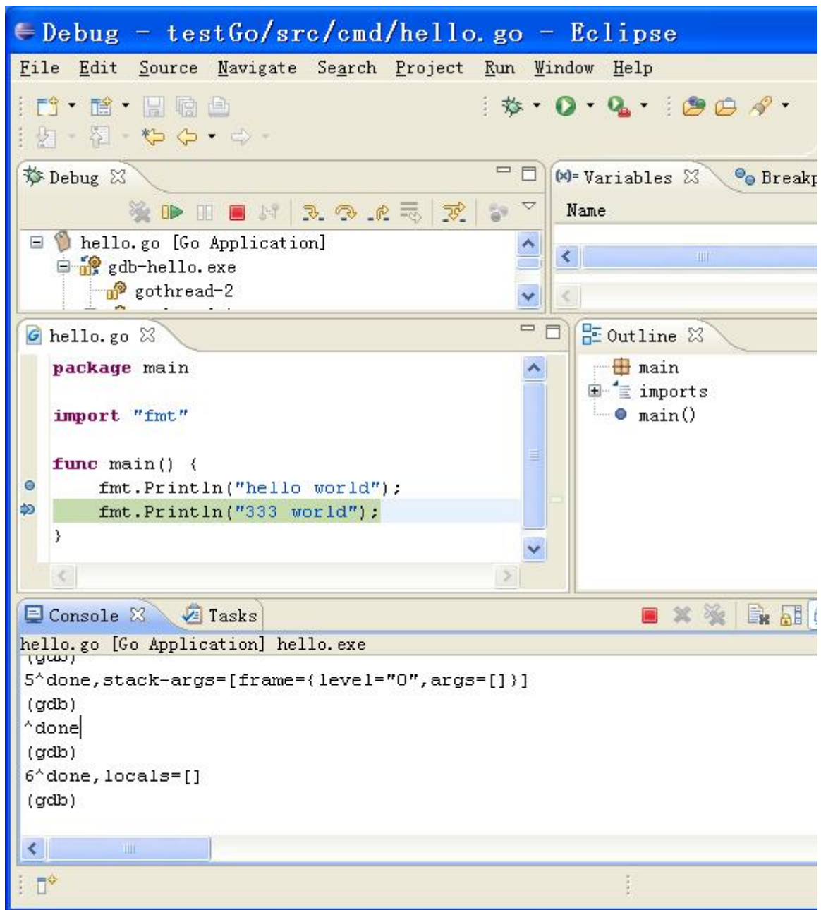
图1.16 调试Go程序
