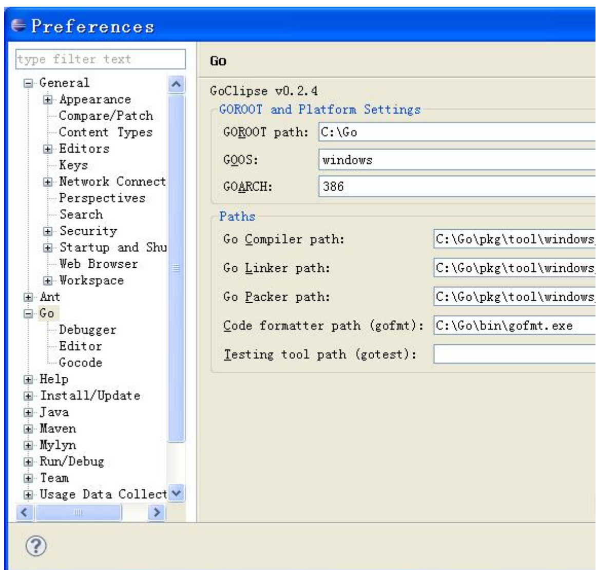
图1.12 设置Go的一些基础信息
