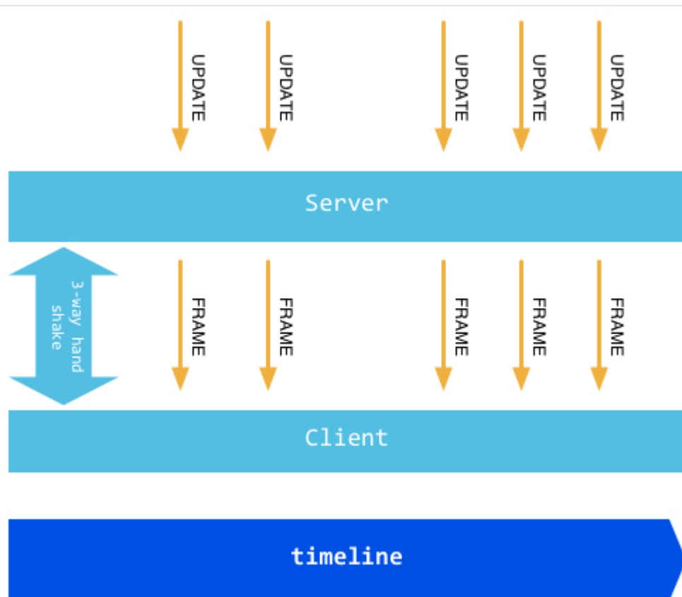
图8.2 WebSocket原理图
