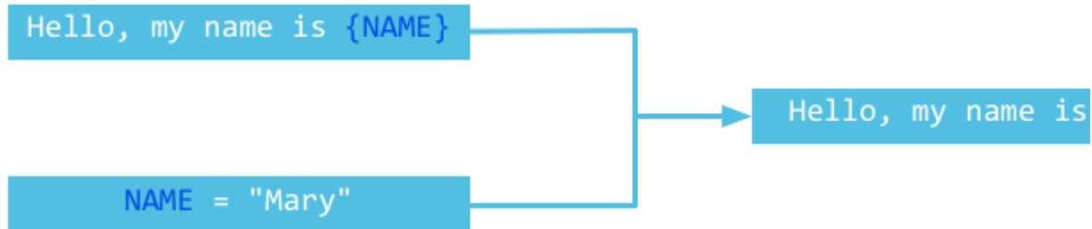
图7.1 模板机制图
