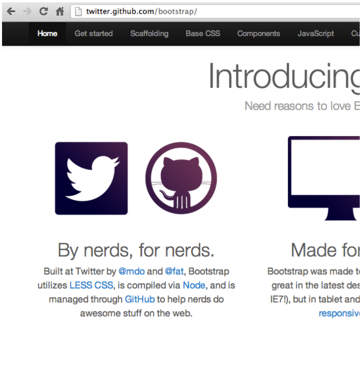
图14.1 bootstrap站点
