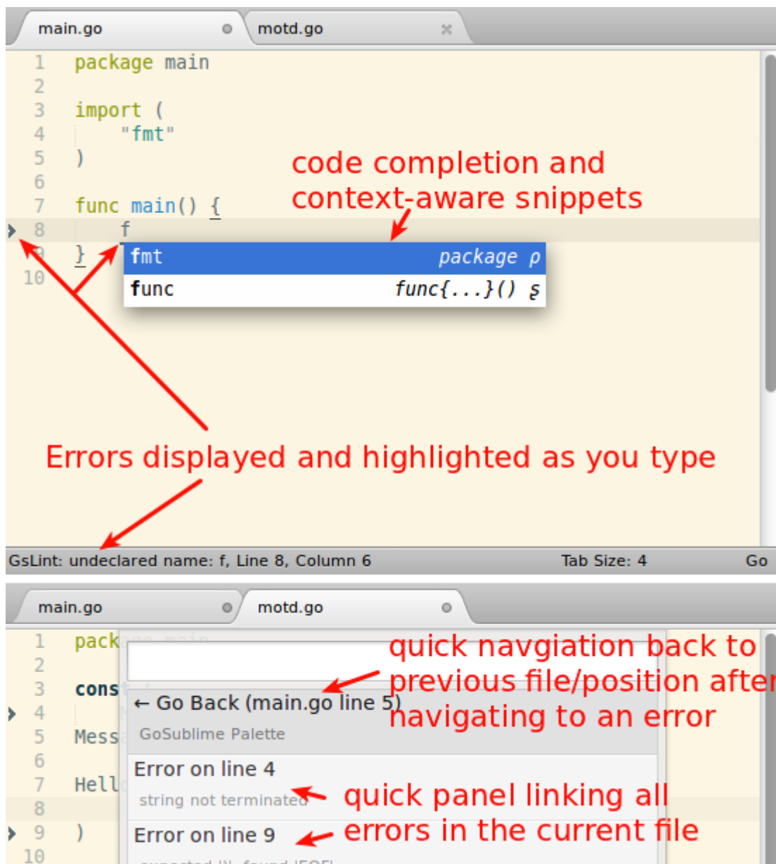
图1.5 sublime自动化提示界面
