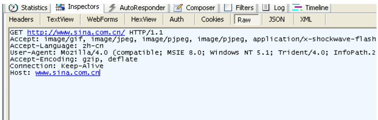
图3.4 fiddler抓取的GET信息
