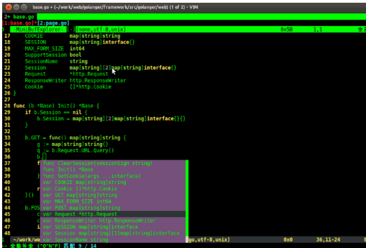
图1.9 VIM编辑器自动化提示Go界面
