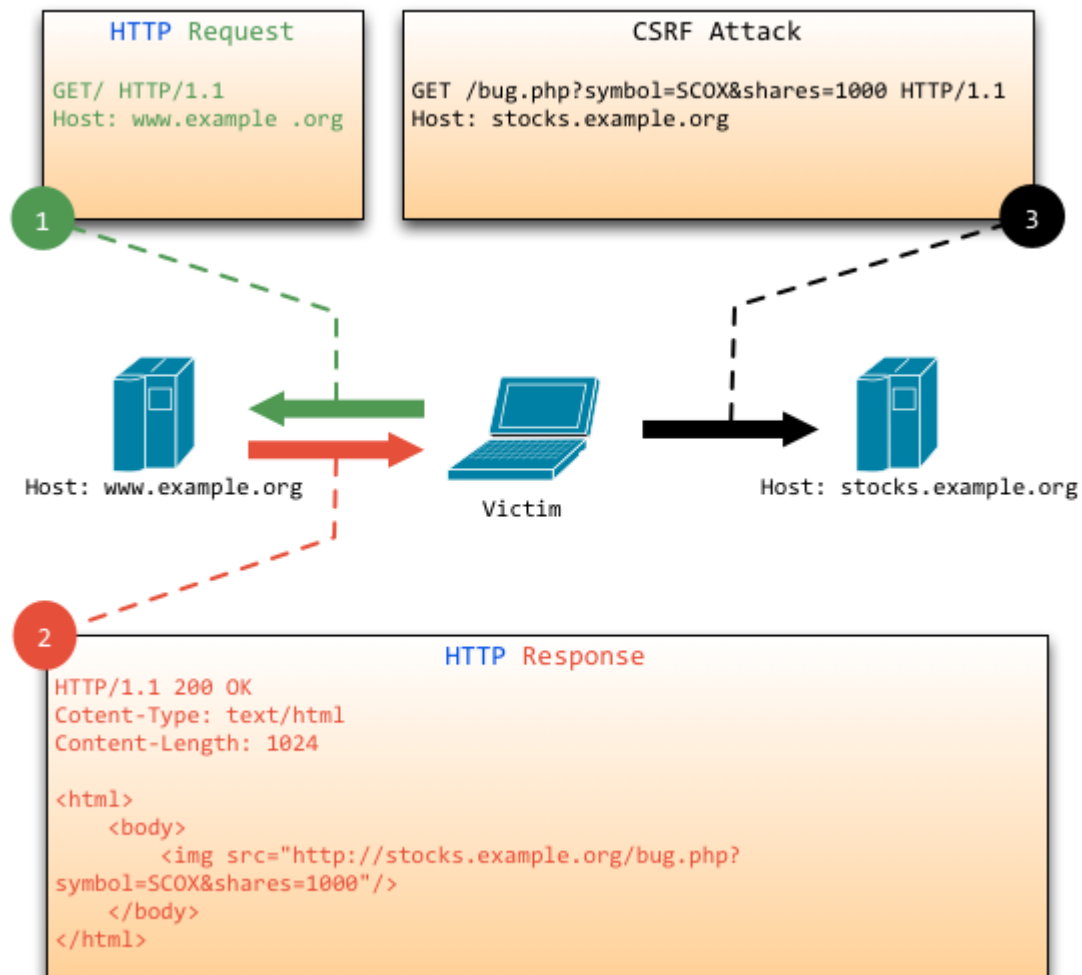
图9.1 CSRF的攻击过程
