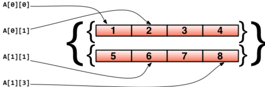
图2.2 多维数组的映射关系
