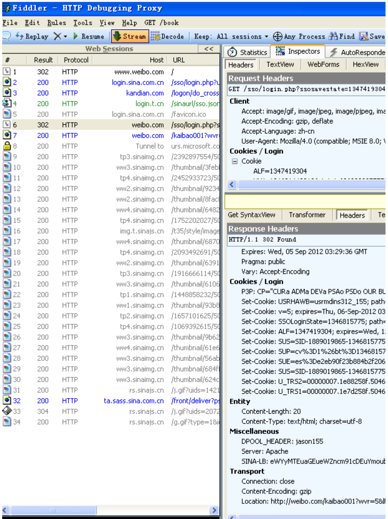
图3.6 访问一次网站的全部请求信息
