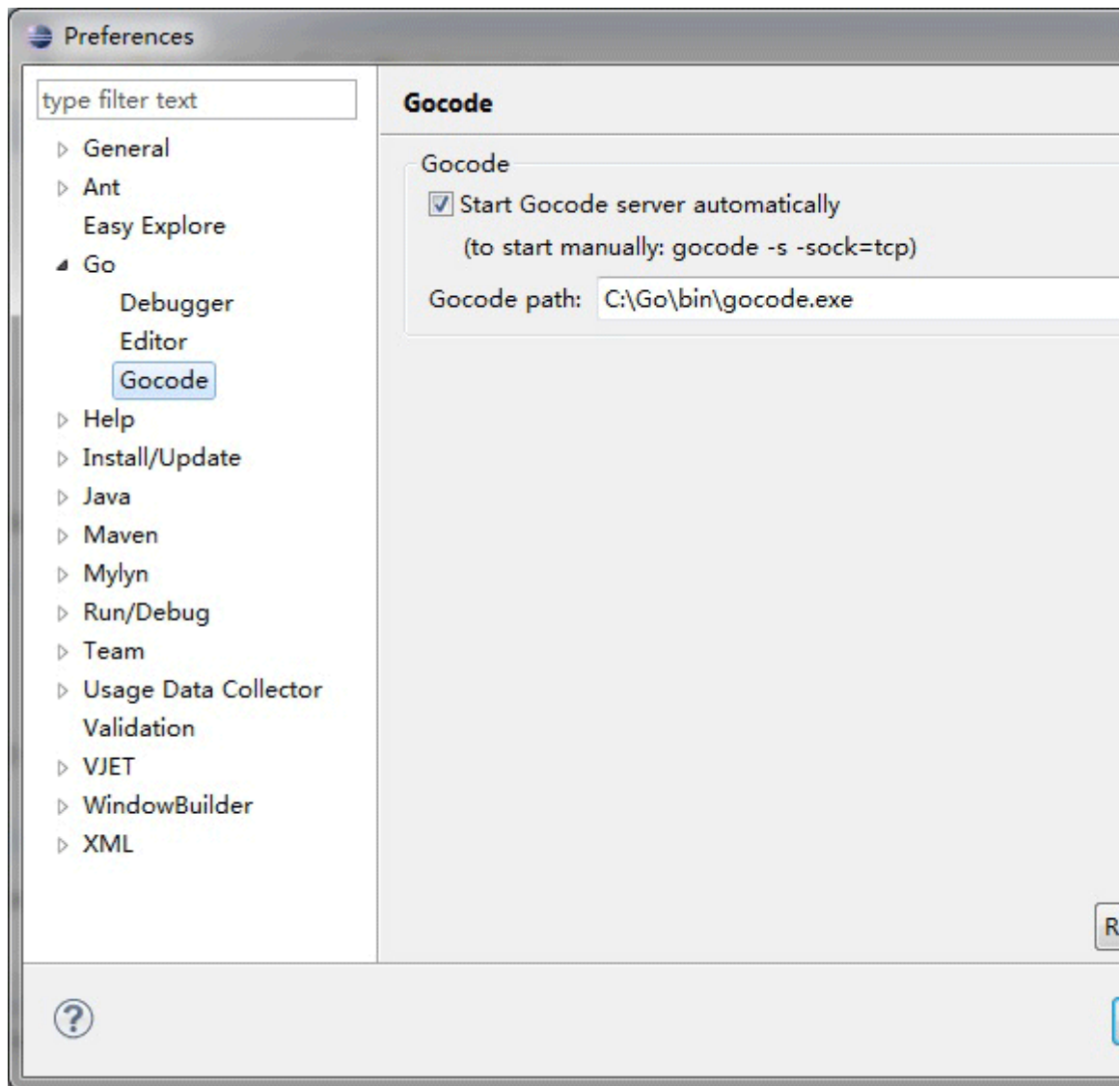
图1.13 设置gocode信息
