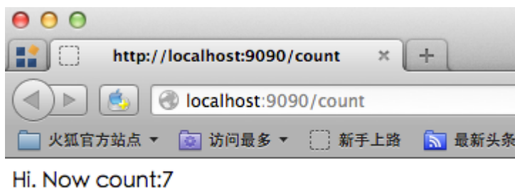
图6.6 模拟cookie
