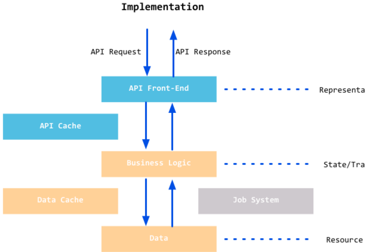
图8.5 REST架构图
