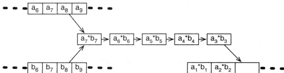
图7-2 多组数乘法的饱和的操作流水线
