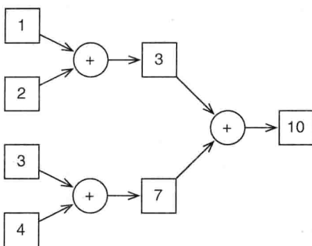
图3-4 (+ (+ 1 2) (+ 3 4))的数据流
