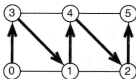
图7-11 三角形带
