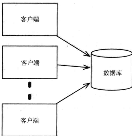
图8-11 传统数据库
