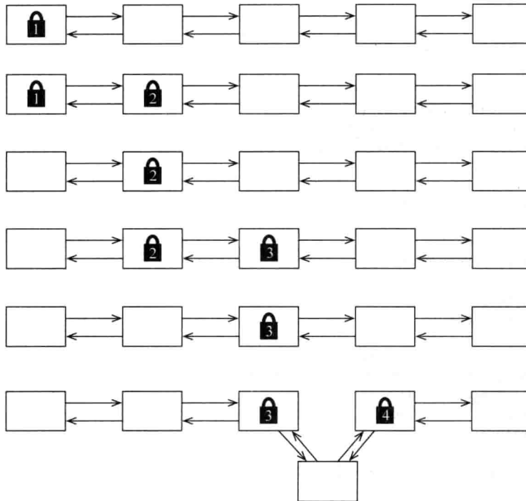
图2-2 交替锁
