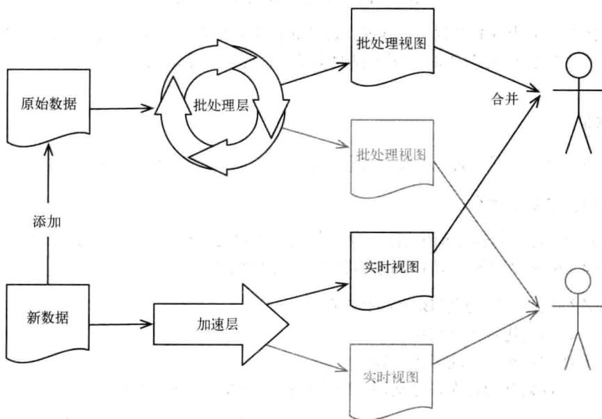
图8-10 Lambda架构
