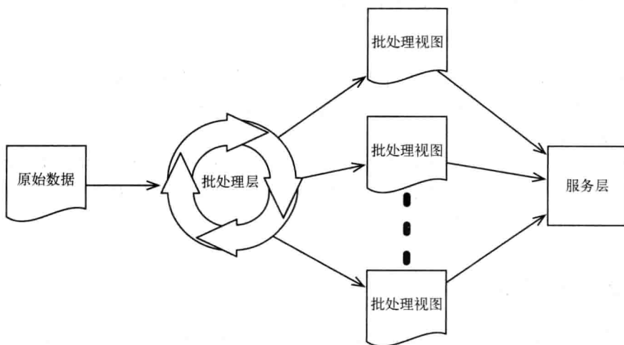
图8-9 数据系统
