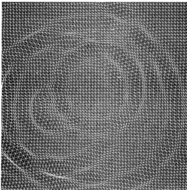
图7-13 水波纹
