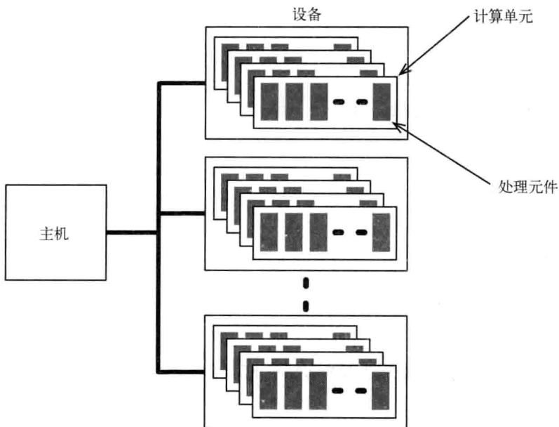
图7-6 OpenCL平台模型
