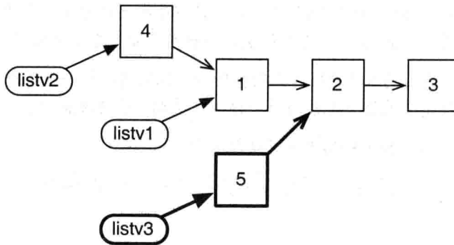
图4-3 listv3在内存中的表现形式
