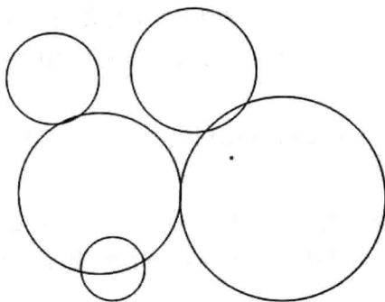
图6-4 衰减的圆
