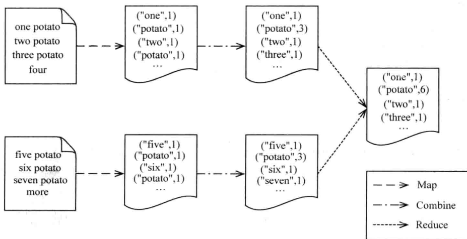
图8-4 使用combiner
