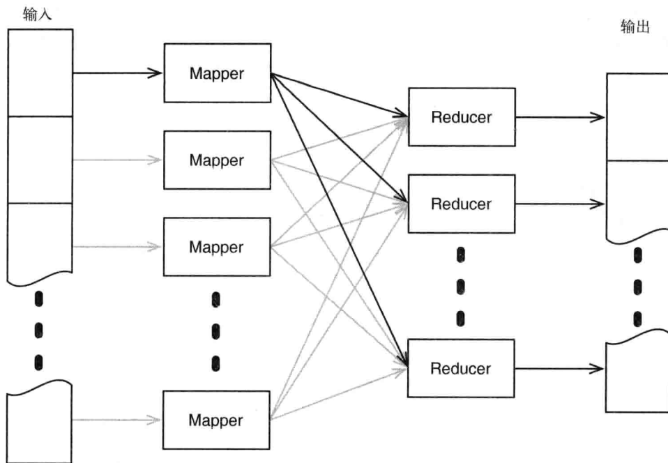
图8-2 Hadoop数据流
