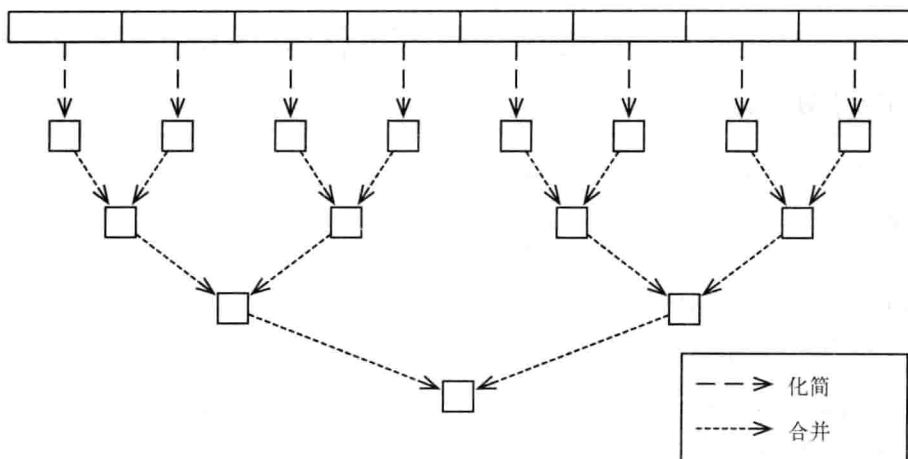
图3-3 fold二叉树
