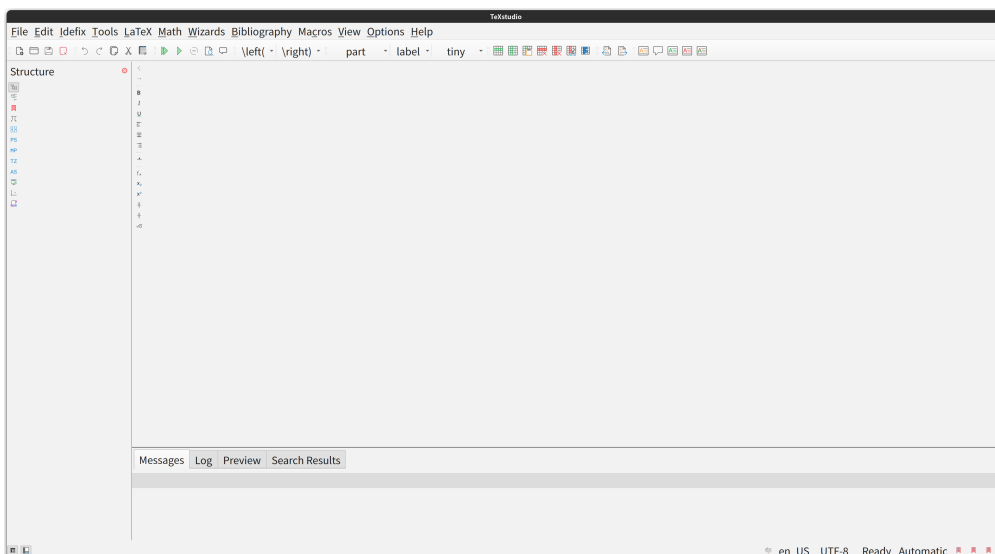
图 1.2 TeXstudio 界面
