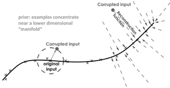
Fig. 15. Denoising auto-encoder.
