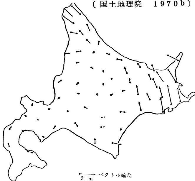
図2 一等三角水平変動ベクトル図 (国土地理院 1970b)
