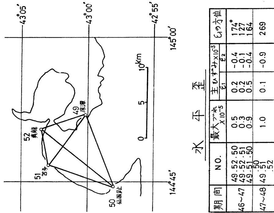
図 1 1 厚岸菱形基線の地震による変化 ( 国土地理院暫定資料 )
