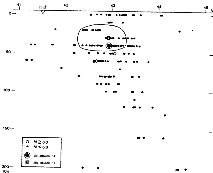
図6.2 北海道東部の地震の南北断面図と今回の地震の余震域
