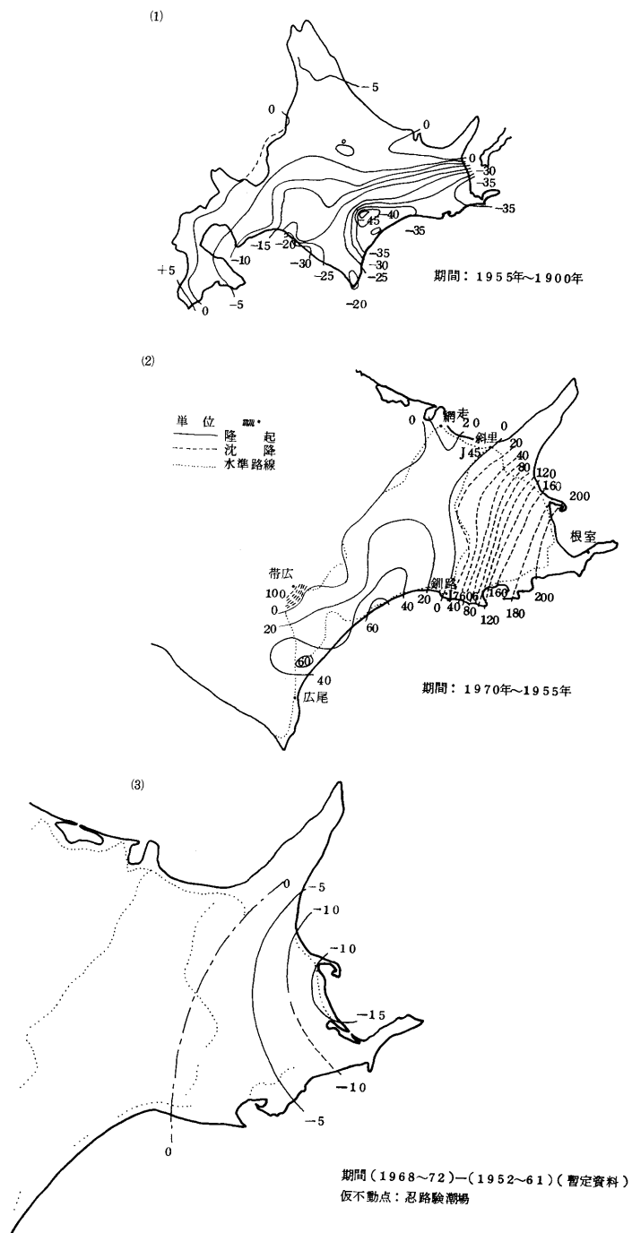
図1 北海道地方上下変動図(国土地理院 1970a, 1971)
