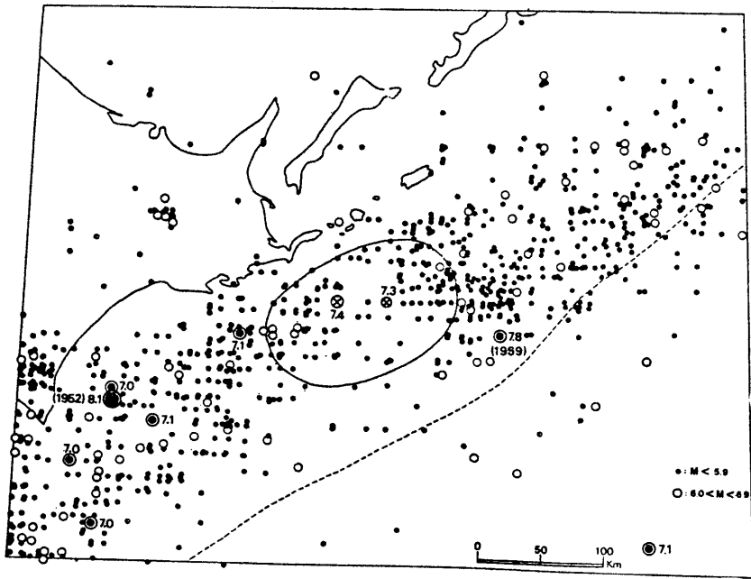
図6.1 1926年以後の地震活動と今回の地震の余震域
