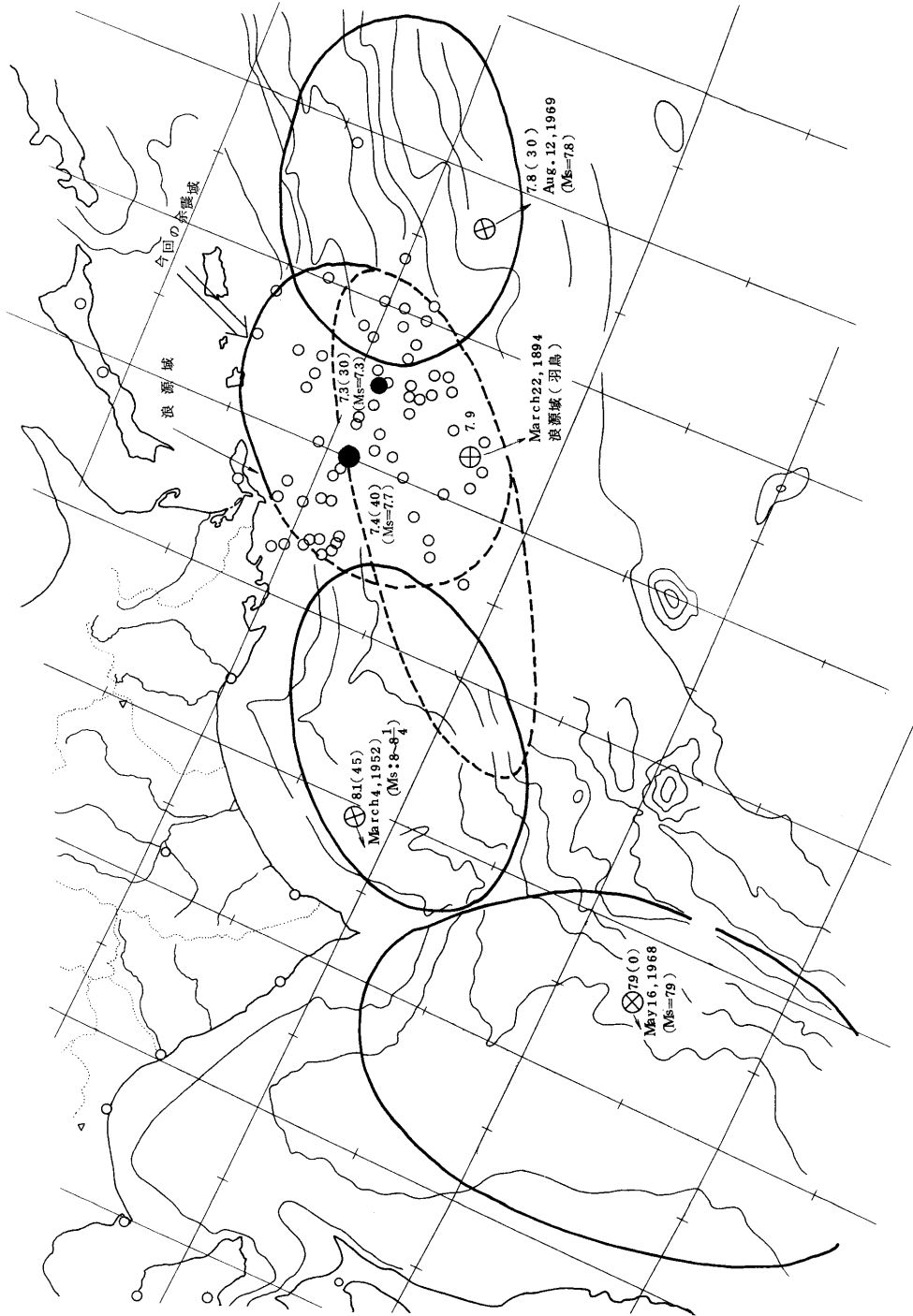
図 1 4 最近の北海道周辺の大地震とその余震域
