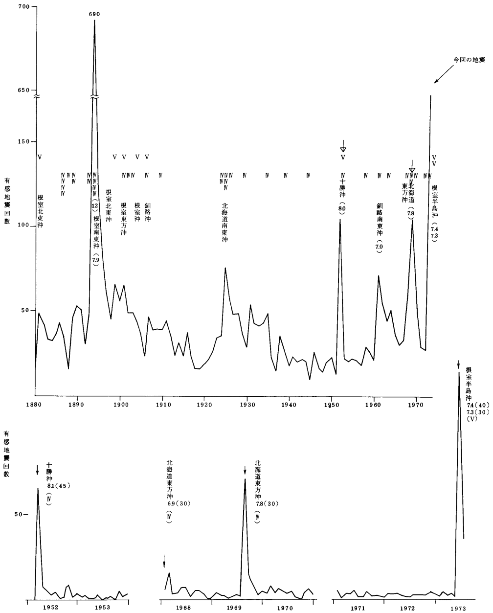
図 1 5. 根室の有感地震回数と大地震の余震回数分布
