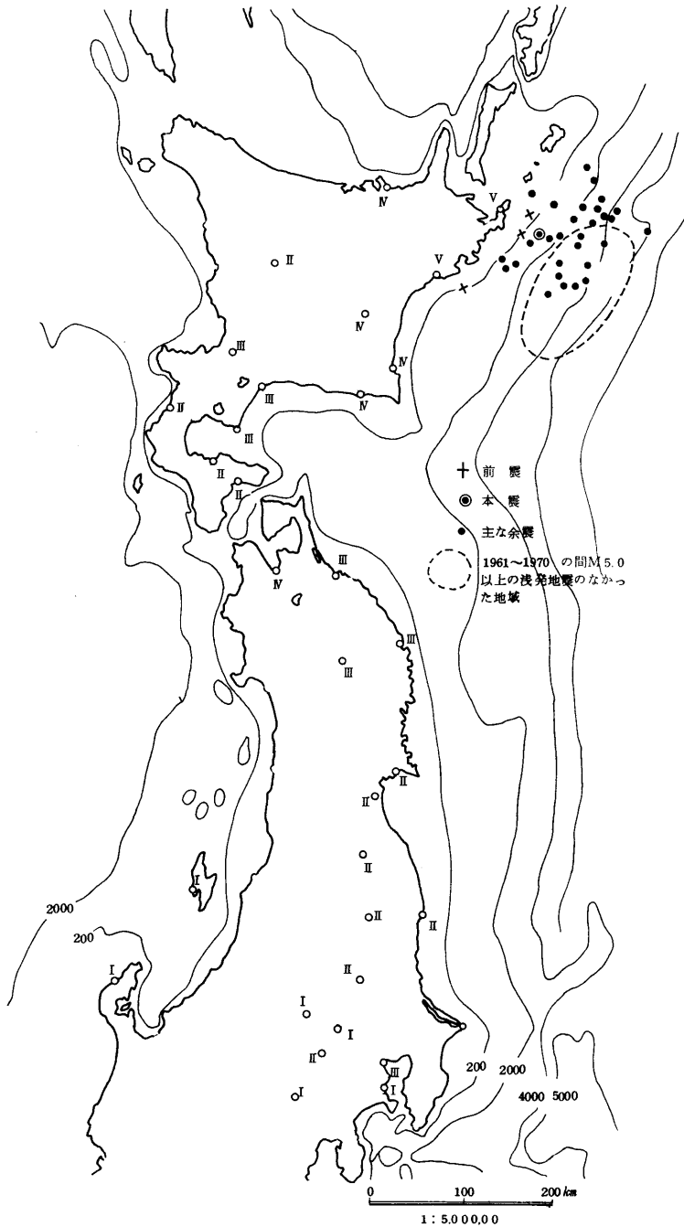
図4 本震の震度分布と前余震の分布(6月中)
