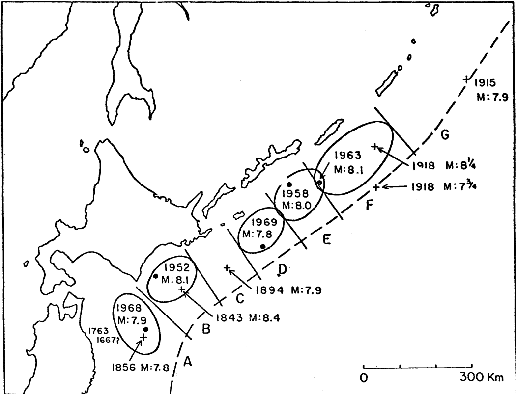
図3 北海道大太平洋沿岸域の過去の大地震と空白域(宇津 1972)
