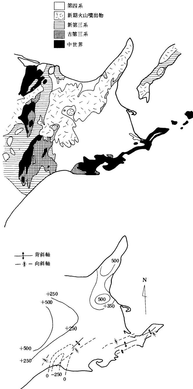
図8 北海道東部の地質（地質調査所1964）と 第四紀の地殻変動（QTMG1969）
