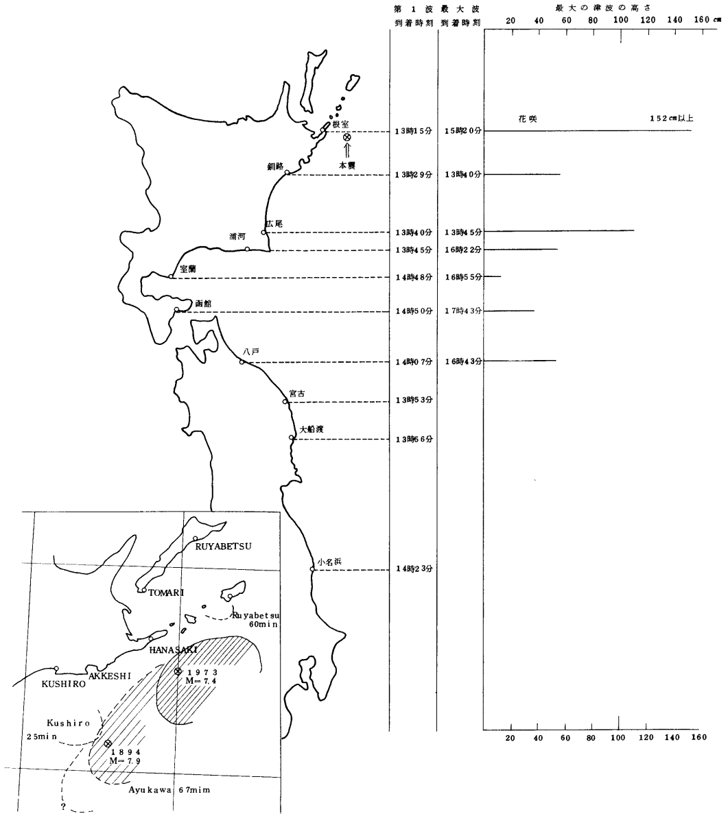
図7 本震による津波（気象庁1973a）と 浪源域（津波研究会による）
