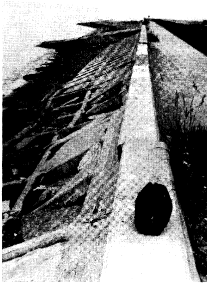
写真7 道路橋被害(1)厚岸大橋
