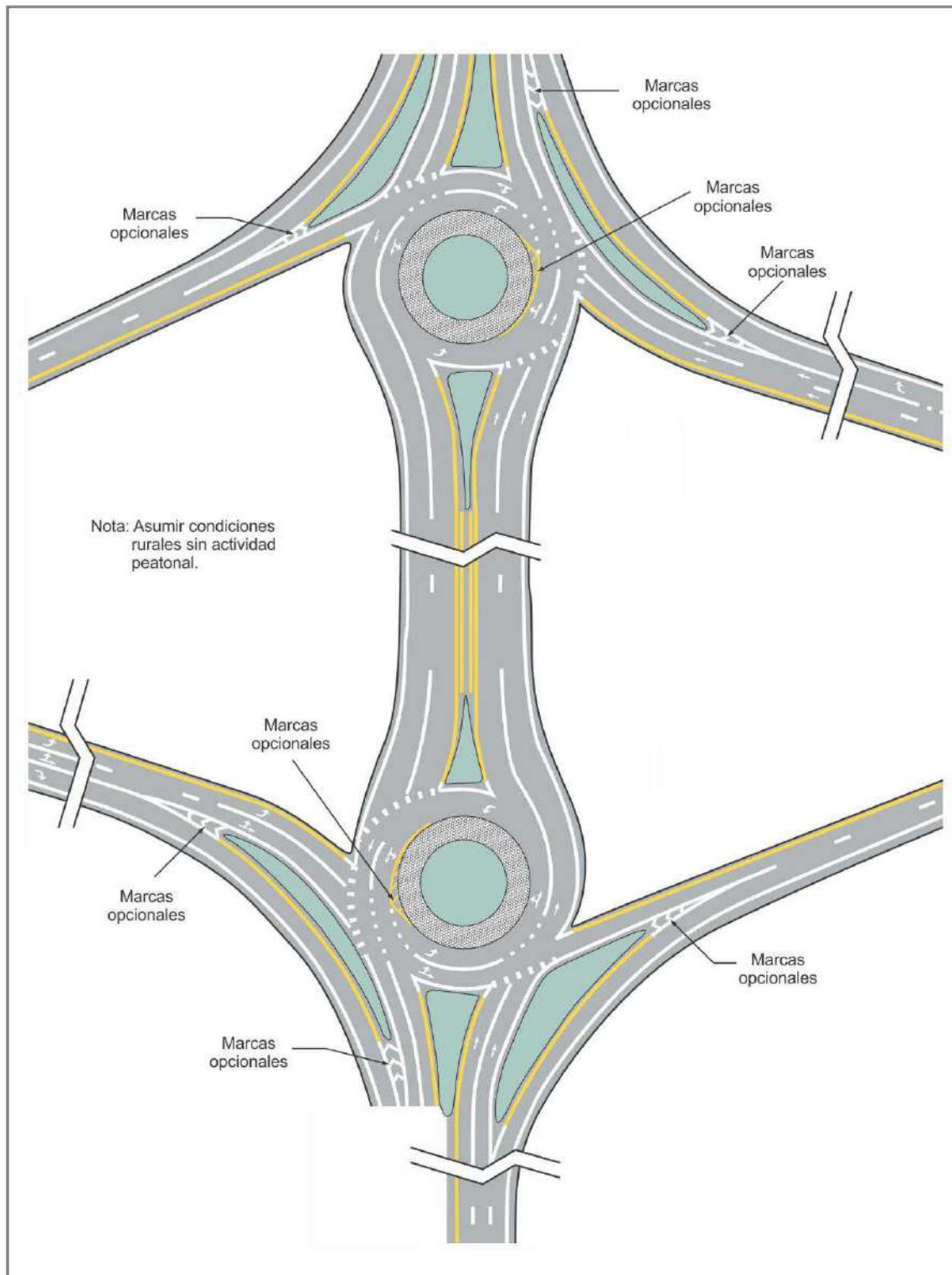
Figura 3.33 Ejemplo de demarcación para una intersección tipo diamante con rotondas o glorietas en los terminales de las rampas
