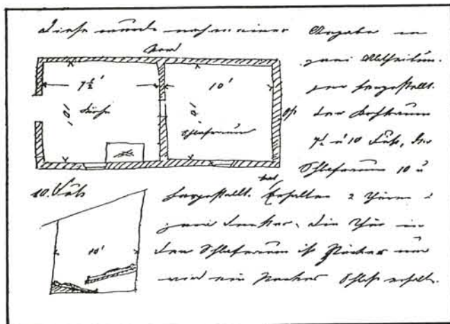
Grundriß des Uraltbaues der Stüdlhütte; Skizze von E. Pegger in einem Brief an Joh. Stüdl. Das Äußere zeigt das Titelbild dieser Schrift.
