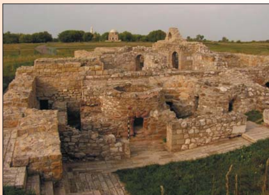
Болгардагы Алтын Урда чоры мунчасы казылмалары.
