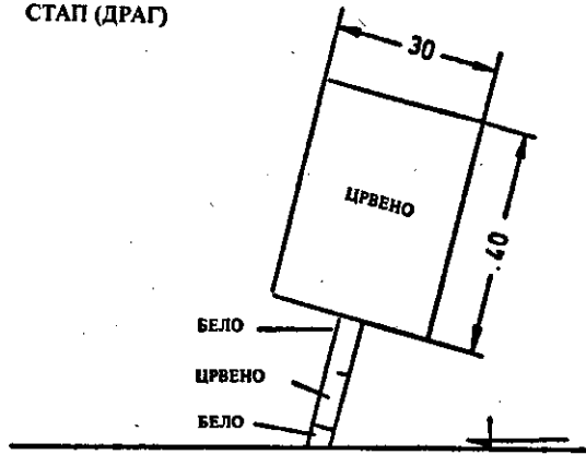
Ноќе: црвени трепкави светилки
