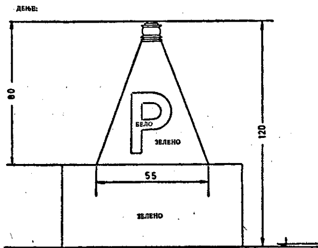
Ноќе: зелени трепкави светилки
