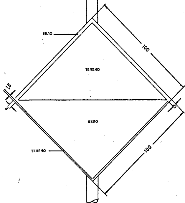
Знаците под Б.2. (фарови на левиот брег) служат за обележување на правецот на пловниот пат односно на брегот и со знаците поставени на водениот пат, тие го обележуваат пловниот пат на местата на кои тој се доближува до левиот брег; тие истовремено служат како ориентациони точки.
