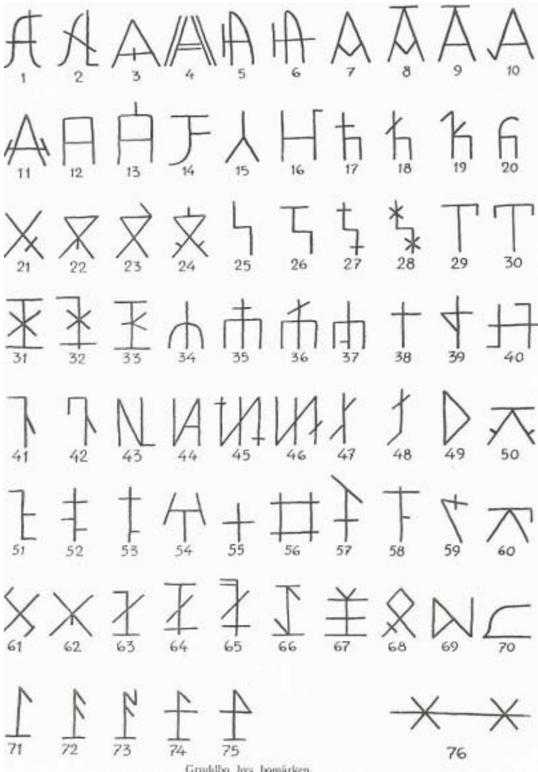
Grundbo-ivs bomärken.
