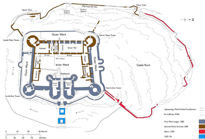
Ffynhonell 16: Cynllun llawr o gastell Harlech
