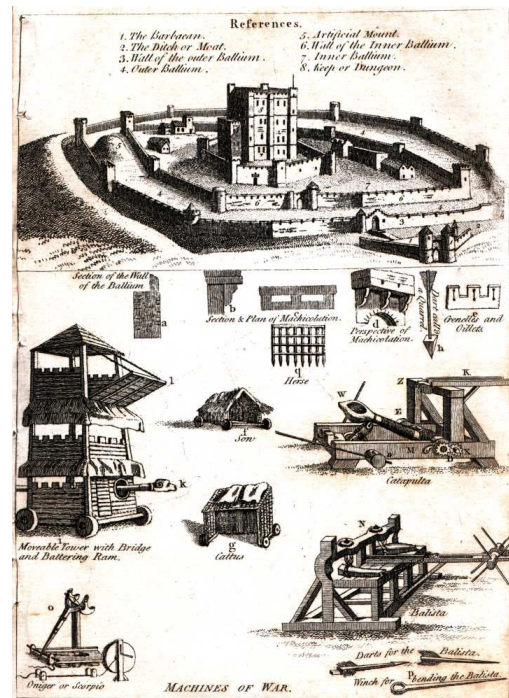
Ffynhonell 14: Peiriannau gwarchae'r Oesoedd Canol
