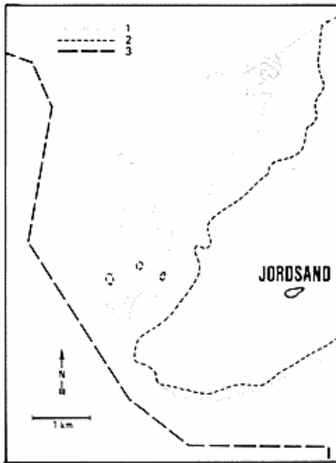
Fig. 16. Der westliche Teil von Jordsands Flak. 1 und 2 Niedrigwasserlinien laut Seekarten (vgl. Seite 21) 3. Dänisch-deutsche Grenze. Fig. 16. Den vestlige del af Jordsands flak. 1 og 2 Lavvandslinier efter søkort (se teksten side 21) 3. Dansk - tysk grænse.
