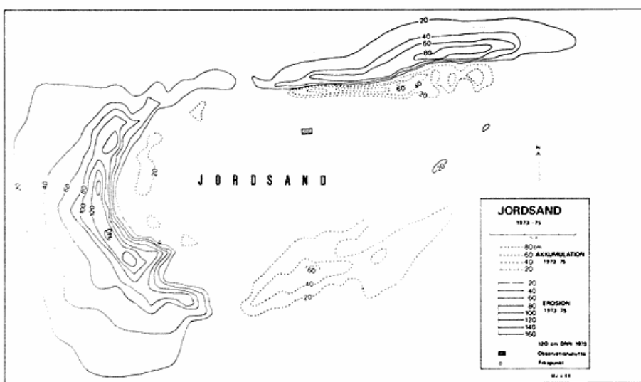
Fig. 10. Akkumulation und Erosion der Insel Jordsand. Fig. 10. Akkumulation og erosion på Jordsand.
