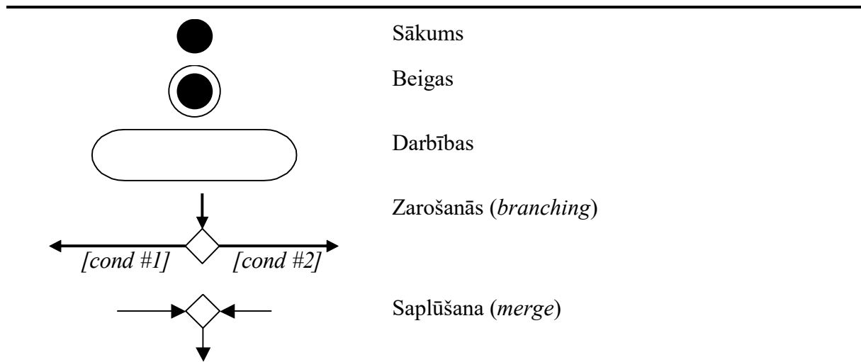
UML aktivitāšu diagrammas konstrukciju apraksts
