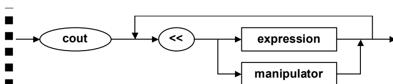
Att. 5.2. Formatēta izvade sintaktiskās diagrammas pierakstā
