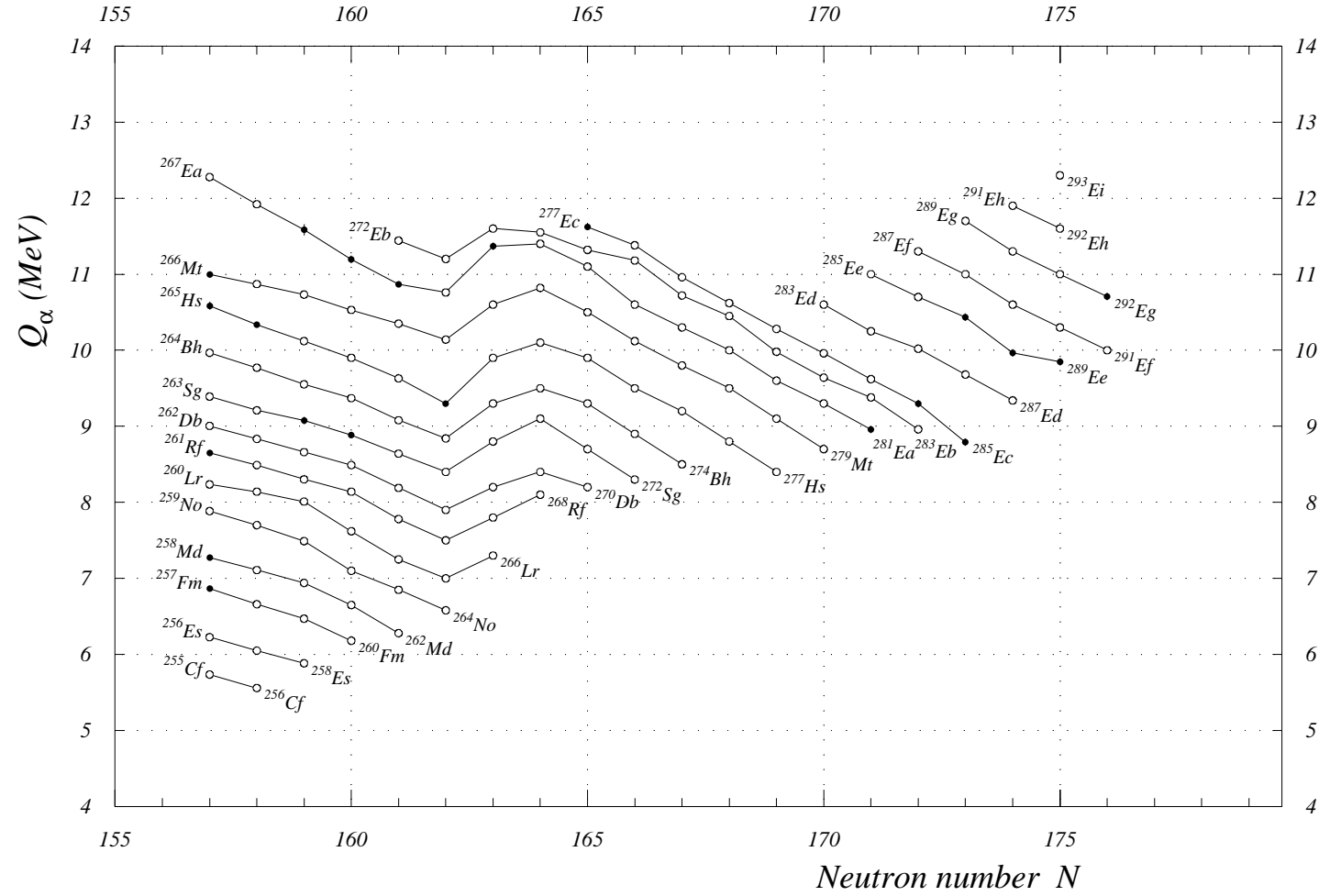
Fig. 26. \alpha -decay energies
